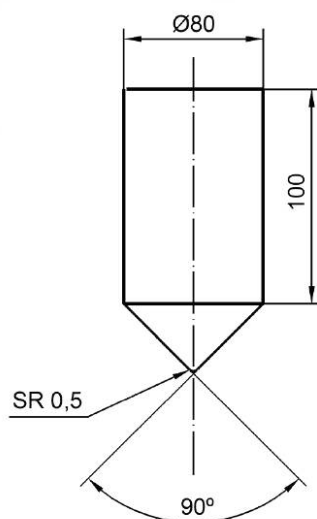
Рисунок 1 — Испытательный конус
