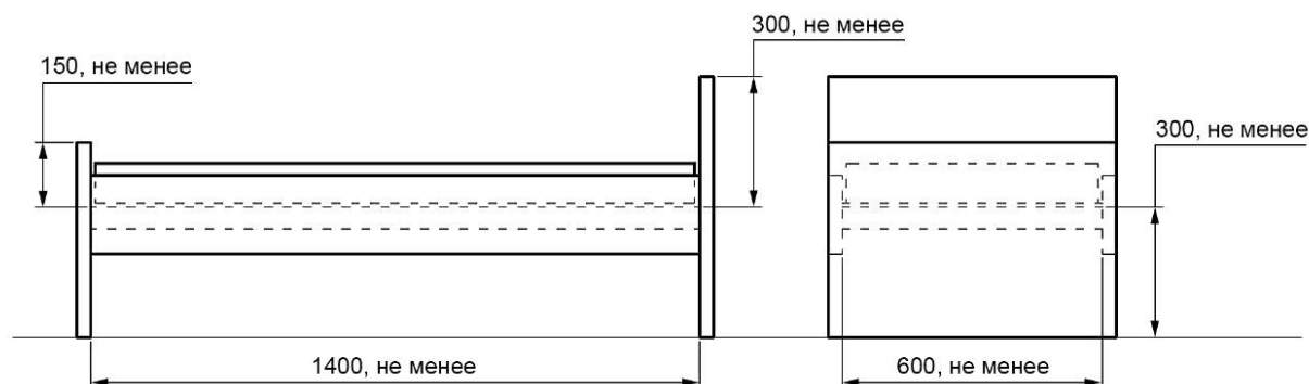
Рисунок 2 — Функциональные размеры детских кроватей типа II
