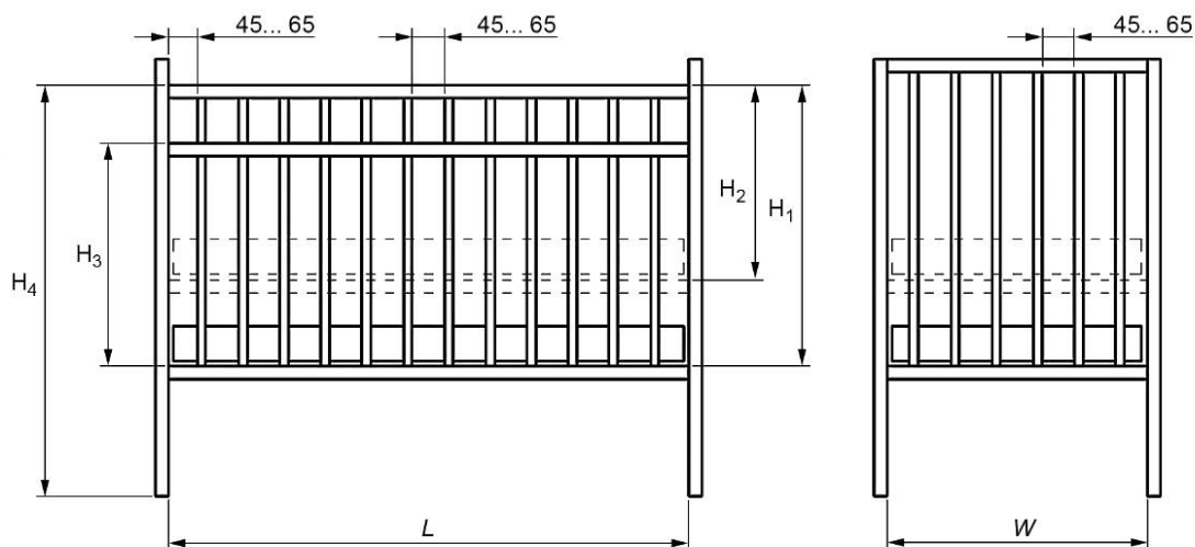
Рисунок 1 — Функциональные размеры детских кроватей типа I
