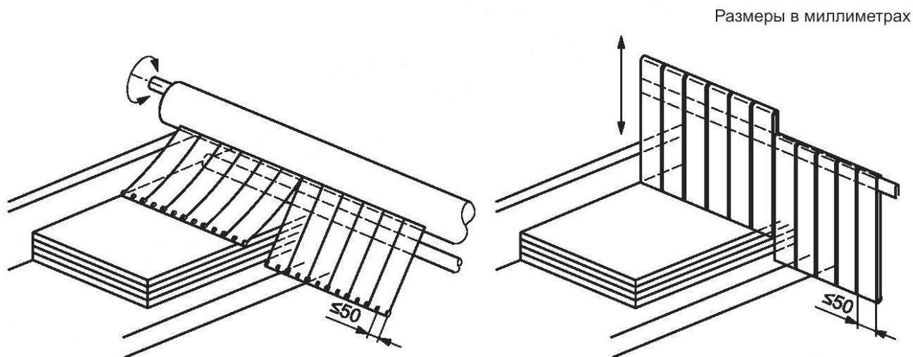
Рисунок 3 — Защитная завеса
