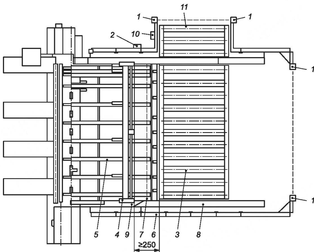
1 — AOPD 1; 2 — орган управления сбросом для подъемной платформы AOPD 1; 3 — подъемная платформа; 4 — толкатель панели; 5 — опора для заготовки станка; 6 — заднее ограждение; 7 — AOPD 2; 8 — предохранительный механический кулачок; 9 — предохранительный выключатель; 10 — держатель для органа управления; 11 — роликовый конвейер
