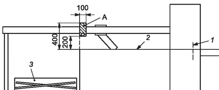
1 — линия резания; 2 — стол станка; 3 — подъемный стол; А — область для AOPD 2
