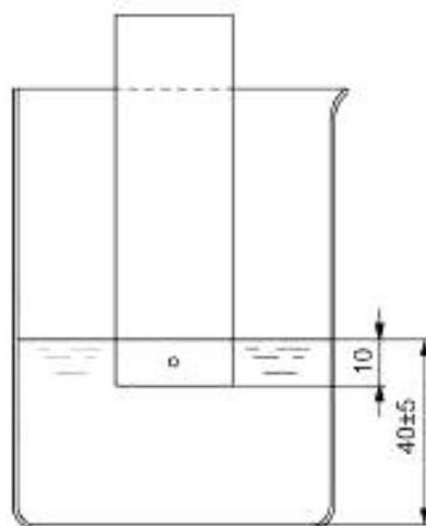
Рисунок 1 — Образец для испытания, помещенный в дистиллированную воду
