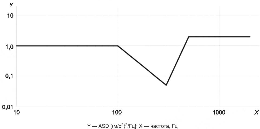
Рисунок 1 — ASD случайной вибрации
