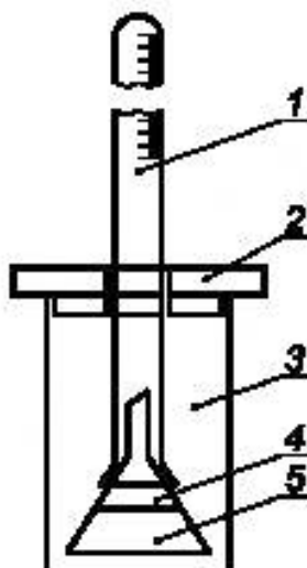
1 — бюретка с делением на 25—50 мл; 2 — крышка из оргстекла; 3 — стеклянный сосуд емкостью 0,5—0,75 л; 4 — стеклянная воронка диаметром 55—65 мм; 5 — испытываемая фольга (рулон высотой 25—30 мм, диаметром 30—40 мм)
