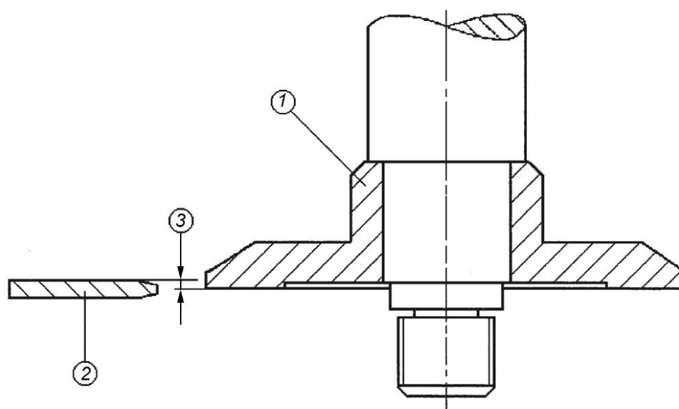
1 — неподвижный фланец дисковой пилы; 2 — расклинивающий нож; 3 — максимальное значение допуска 0,2 мм
