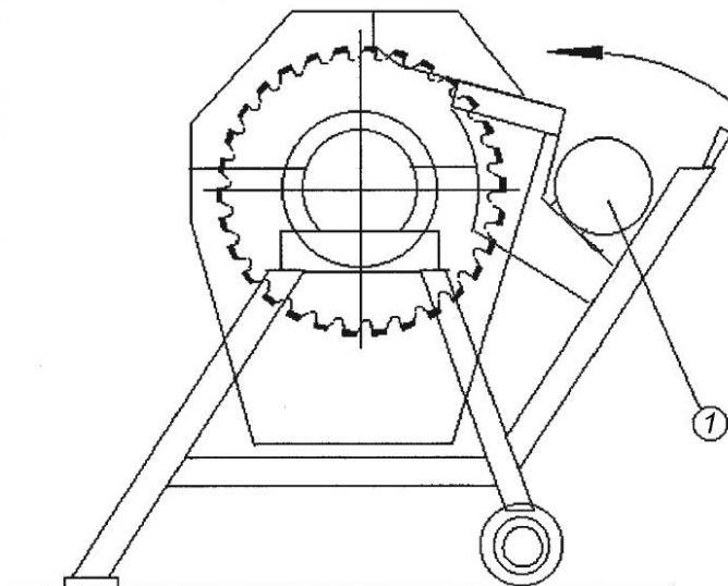
1 — древесина диаметром 70 мм
