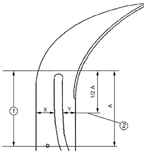
Рисунок 15 — Ширина расклинивающего ножа в области крепления
