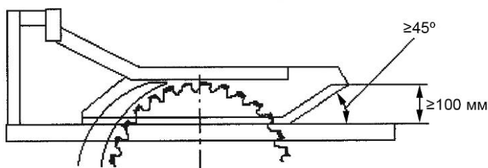
Рисунок 29 а) — Регулируемое защитное ограждение дисковой пилы с заборной частью
