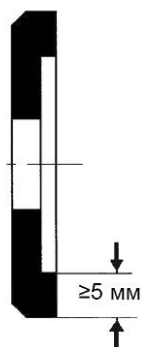
Рисунок 8 — Пример фланца дисковой пилы
