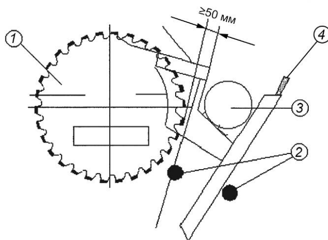
1 — дисковая пила максимального диаметра; 2 — упоры; 3 — заготовка; 4 — ручка
