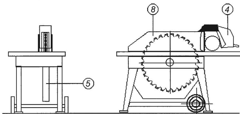
Рисунок 4 б) — Комбинированный лесопильный станок с роликовым столом/настольный круглопильный станок в режиме эксплуатации настольного лесопильного станка
