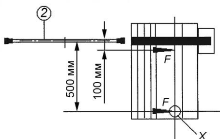
Рисунок А.1 — Испытание на сопротивление скручиванию поворотного стола
