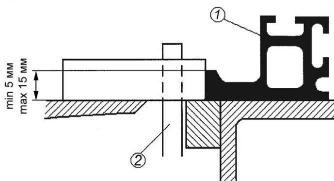
1 — направляющая; 2 — пила
