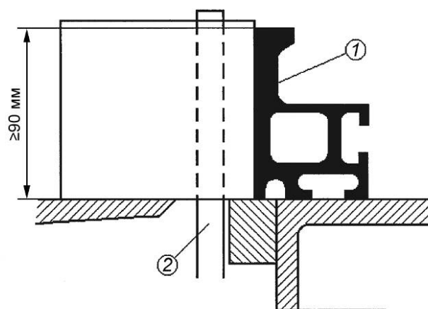
1 — направляющая; 2 — пила
