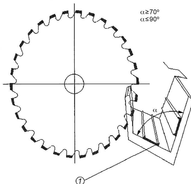
Рисунок 17 — Деталь опорной поверхности поворотного стола
