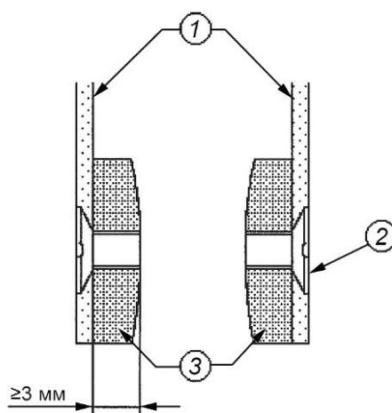
1 — боковые стенки; 2 — крепежные винты; 3 — выступы
