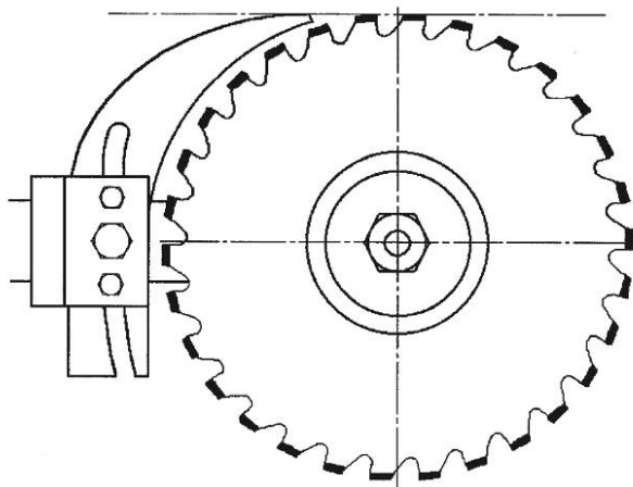
Рисунок 11 — Регулировка высоты раскливающего ножа
