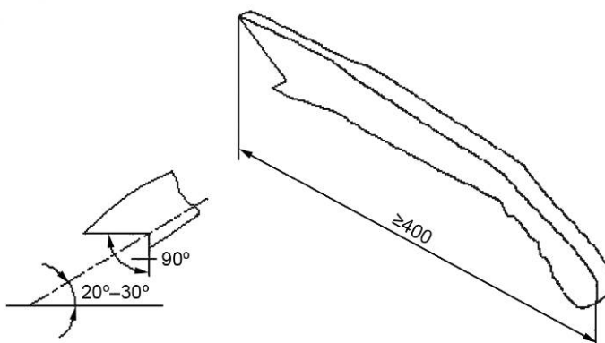
Рисунок 5 б) — Пример толкателя
