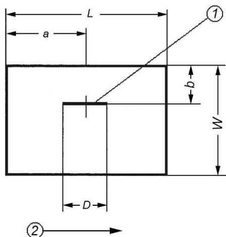
Рисунок F.1 — Минимальные размеры стола для комбинированных лесопильных и настольных круглопильных станков
