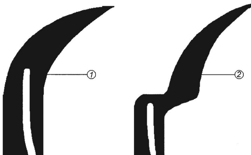
1 — пример допустимой формы расклинивающего ножа; 2 — пример недопустимой формы расклинивающего ножа
