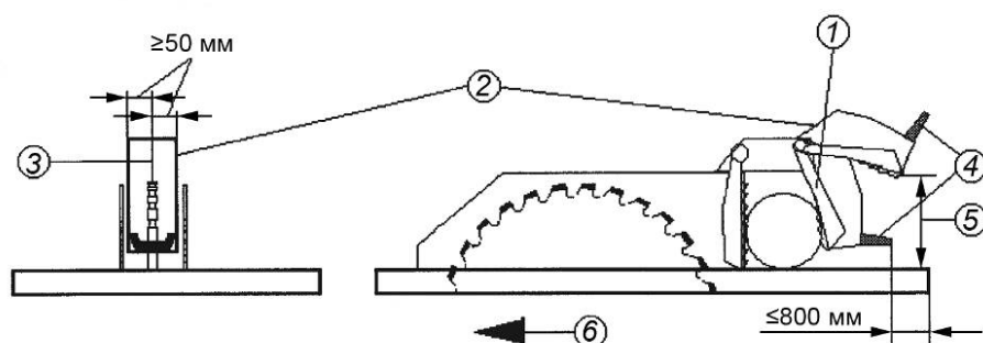
1 — устройство зажима заготовки; 2 — защитное/задерживающее устройство; 3 — линия распила; 4 — ручка; 5 — верхнее нейтральное положение X; 6 — направление распиливания
