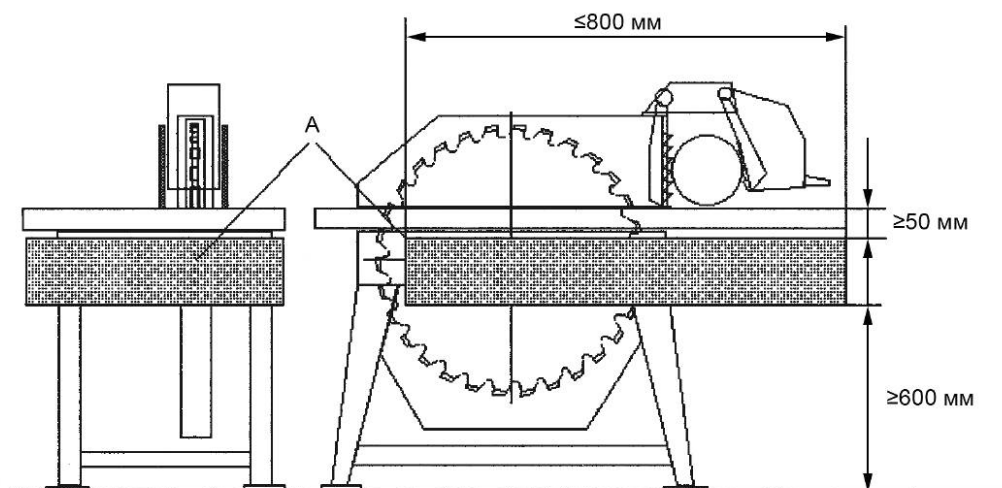
Рисунок 7 — Органы управления для лесопильных станков с роликовым столом
