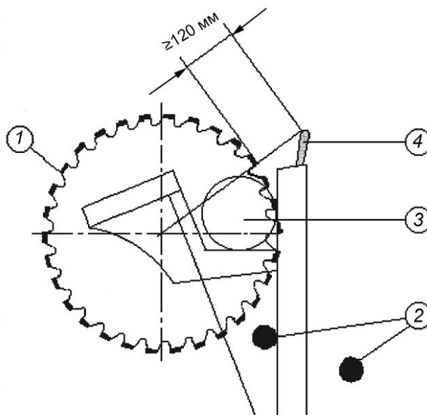
1 — дисковая пила максимального диаметра; 2 — упоры; 3 — заготовка; 4 — ручка
