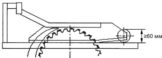
Рисунок 29 b) — Регулируемое защитное ограждение дисковой пилы с направляющими роликами
