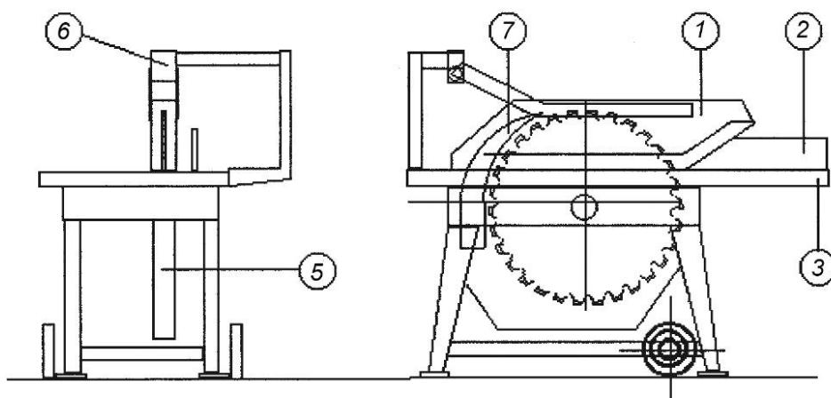
Рисунок 4 а) — Комбинированный лесопильный станок с роликовым столом/настольный круглопильный станок в режиме эксплуатации настольного круглопильного станка
