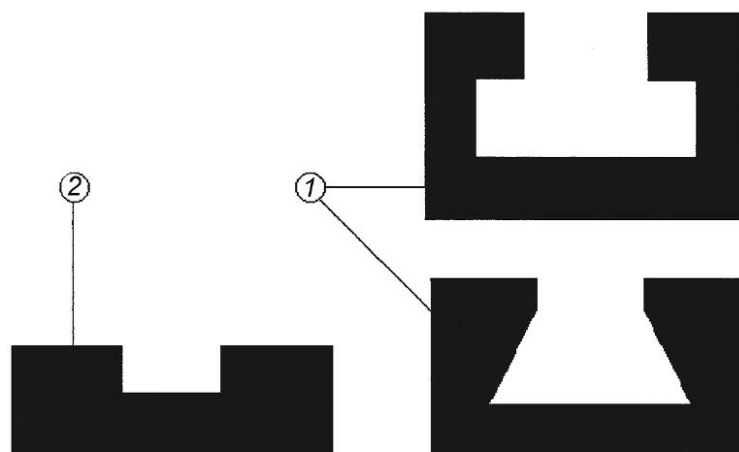
1 — допустимая форма; 2 — недопустимая форма
