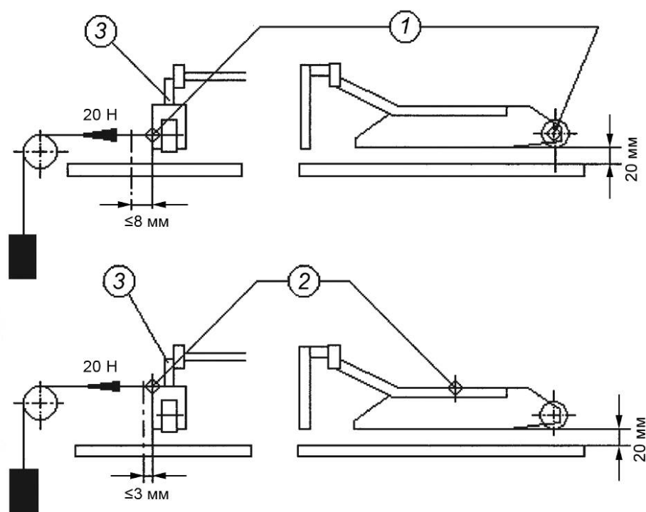
Рисунок G.2 — Испытание на жесткость защитного ограждения
