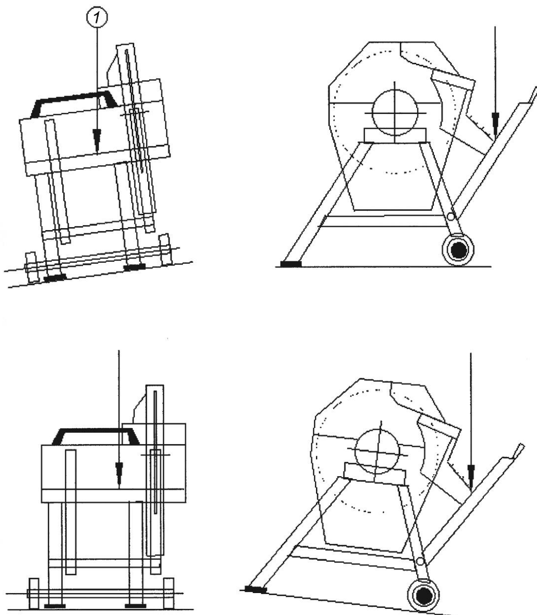
Рисунок А.3 — Испытание на устойчивость станков с поворотным столом
