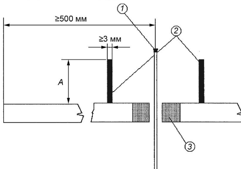
1 — дисковая пила; 2 — упоры заготовки; 3 — вставка стола; A — \geq 80 % максимальной высоты распиливания
