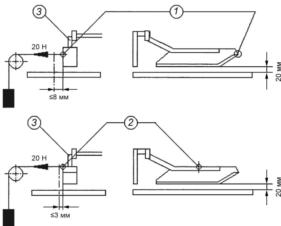
Рисунок G.1 — Испытание на жесткость защитного ограждения
