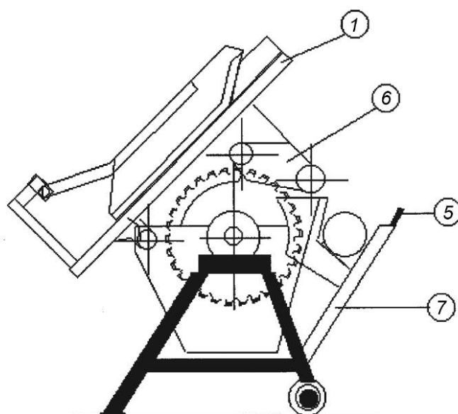
Рисунок 3 б) — Комбинированный лесопильный станок с откидным столом/настольный круглопильный станок в режиме эксплуатации лесопильного станка
