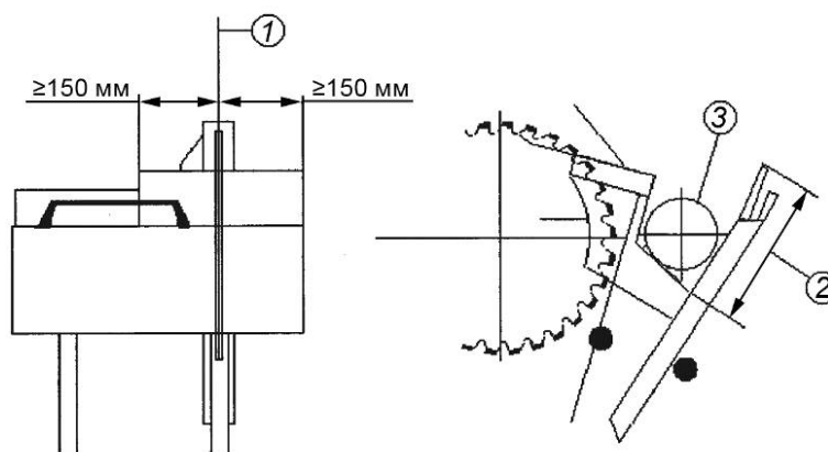
Рисунок 25 — Детальное изображение защиты дисковой пилы лесопильных станков с поворотным столом
