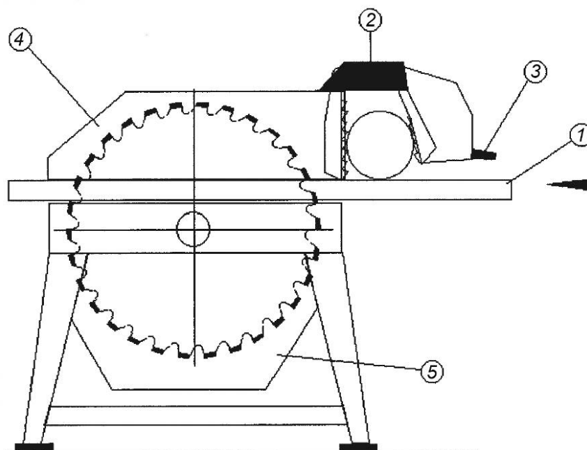
Рисунок 1 — Образец лесопильного станка с поворотным столом
