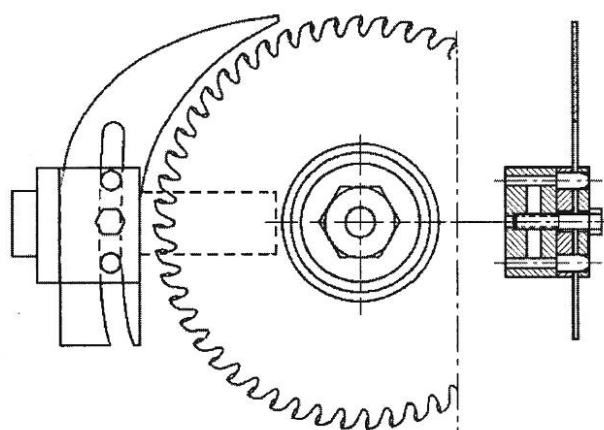
Рисунок 16 — Пример крепления расклинивающего ножа
