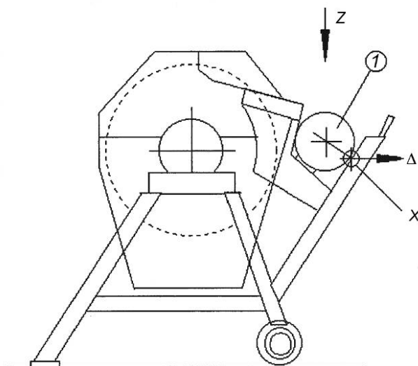
ВИД Z
