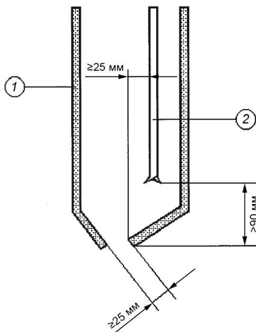
1 — защитное ограждение дисковой пилы; 2 — дисковая пила
