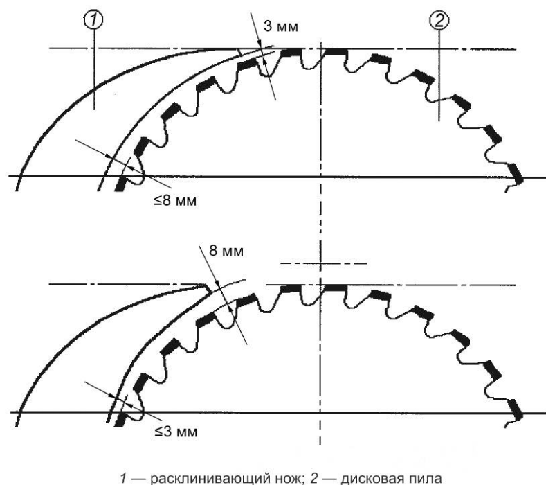
Рисунок 12 — Размеры при установке раскливающего ножа
