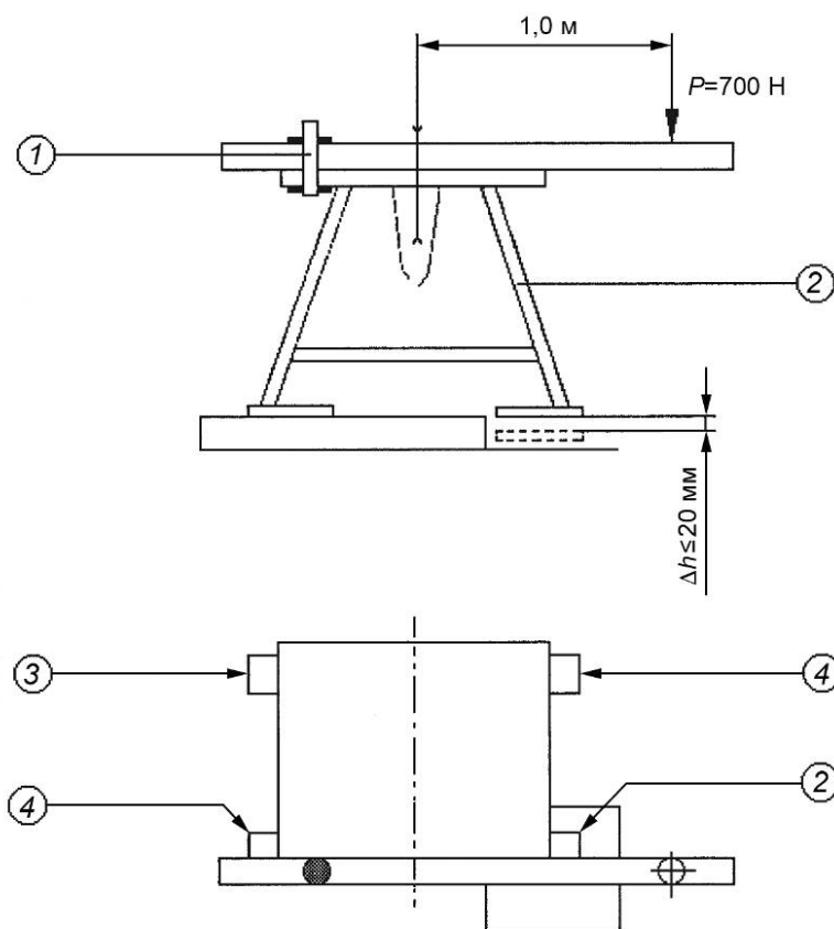
Рисунок А.2 — Испытание на жесткость комбинированных лесопильных и настольных круглопильных станков в режиме работы настольного круглопильного станка
