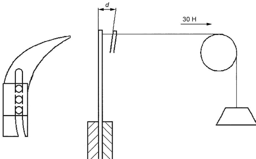
Рисунок D.1 — Испытание расклинивающего ножа на боковую устойчивость
