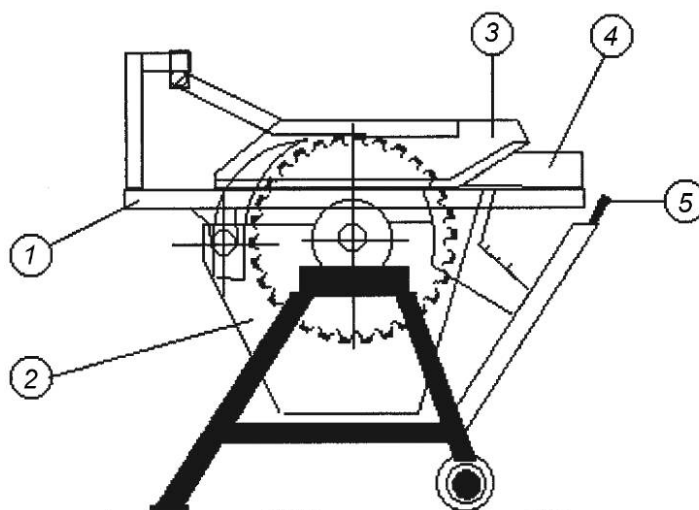
Рисунок 3 а) — Комбинированный лесопильный станок с поворотным столом/настольный круглопильный станок в режиме эксплуатации настольного круглопильного станка
