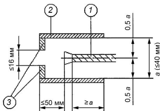
Рисунок 25 б) — Детальное изображение защиты дисковой пилы при открытом элементе дисковой пилы в процессе распиливания
