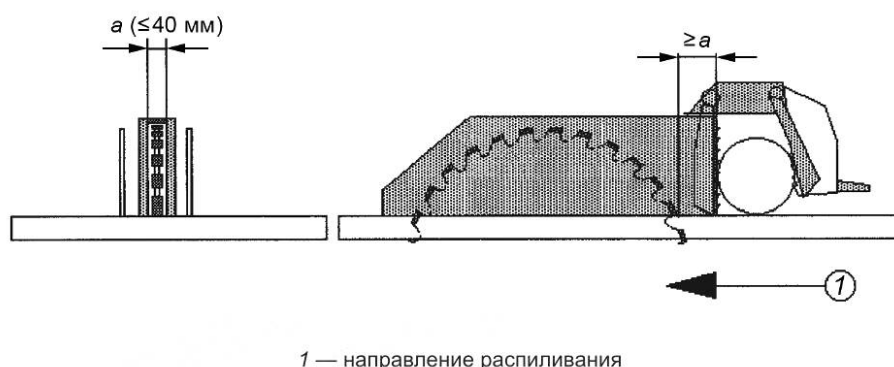
Рисунок 27 — Детальное изображение неподвижного защитного ограждения над роликовым столом
