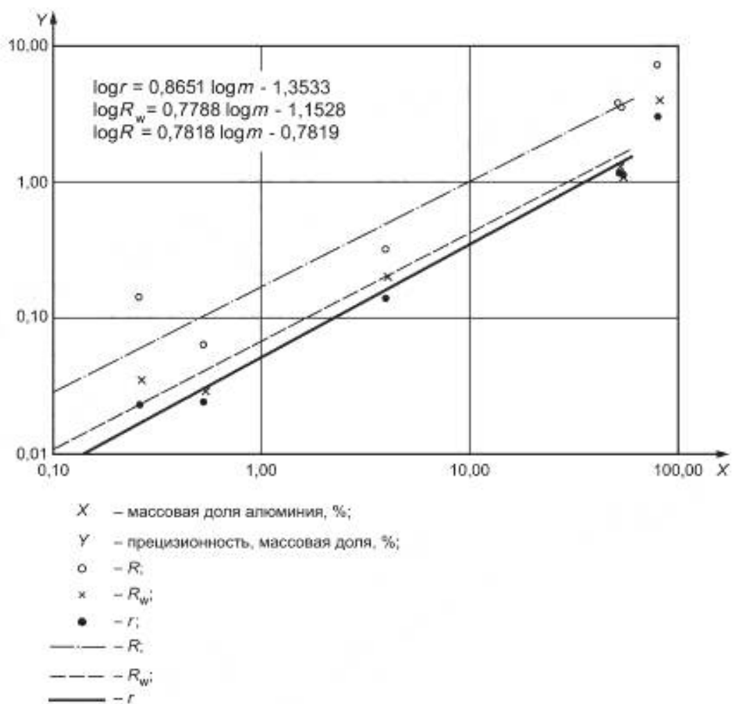
Рисунок С.3 — Данные прецизионности для определения алюминия
