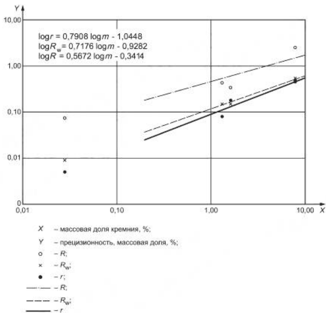
Рисунок С.5 — Данные прецизионности для определения кремния
