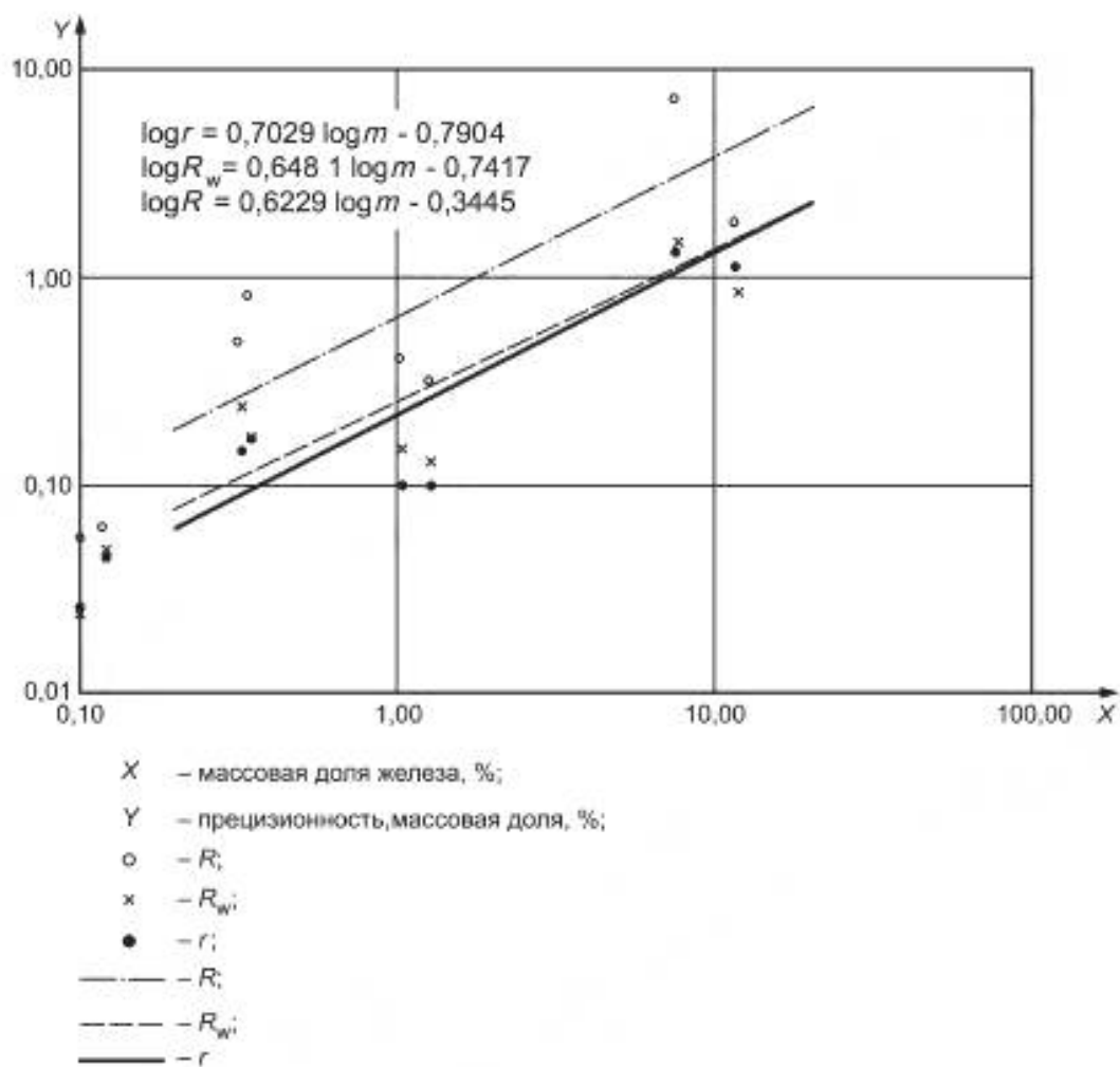
Рисунок С.4 — Данные прецизионности для определения железа
