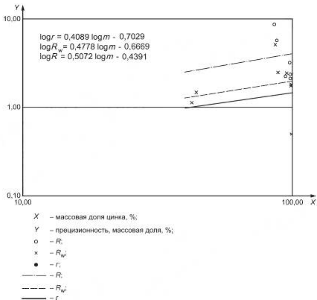
Рисунок С.2 — Данные прецизионности для определения цинка
