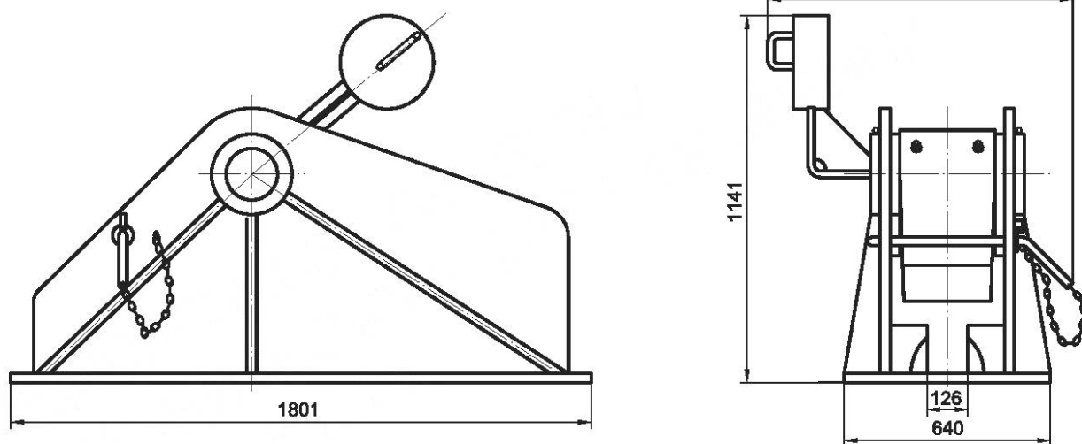
Рисунок А.3 — Цепной стопор с язычком с SWL = 350 т
