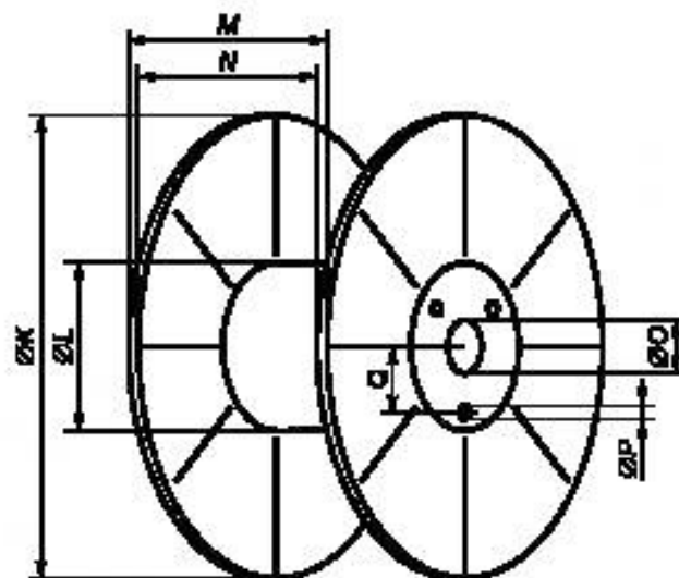
Рисунок 2 — Размер катушки
