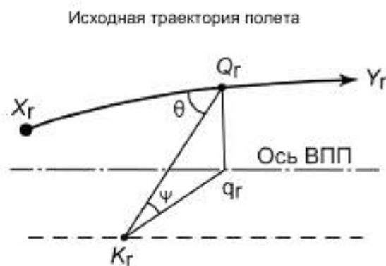
Рисунок 4 — Участки измеренной и исходной траекторий полета на оси ВПП
