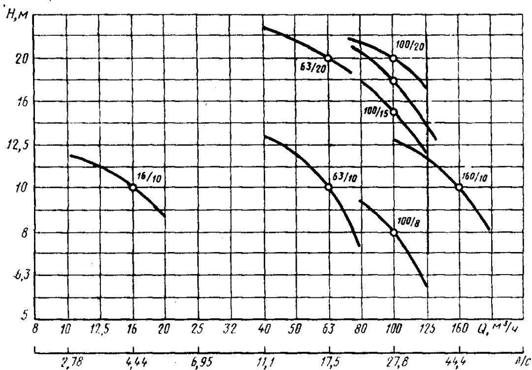
Поле Q-H
