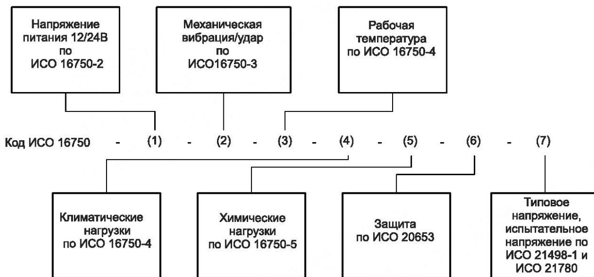
Рисунок 1 — Присвоение кода
