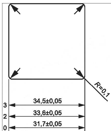
Рисунок 3 — Горизонтальное сечение A-A
