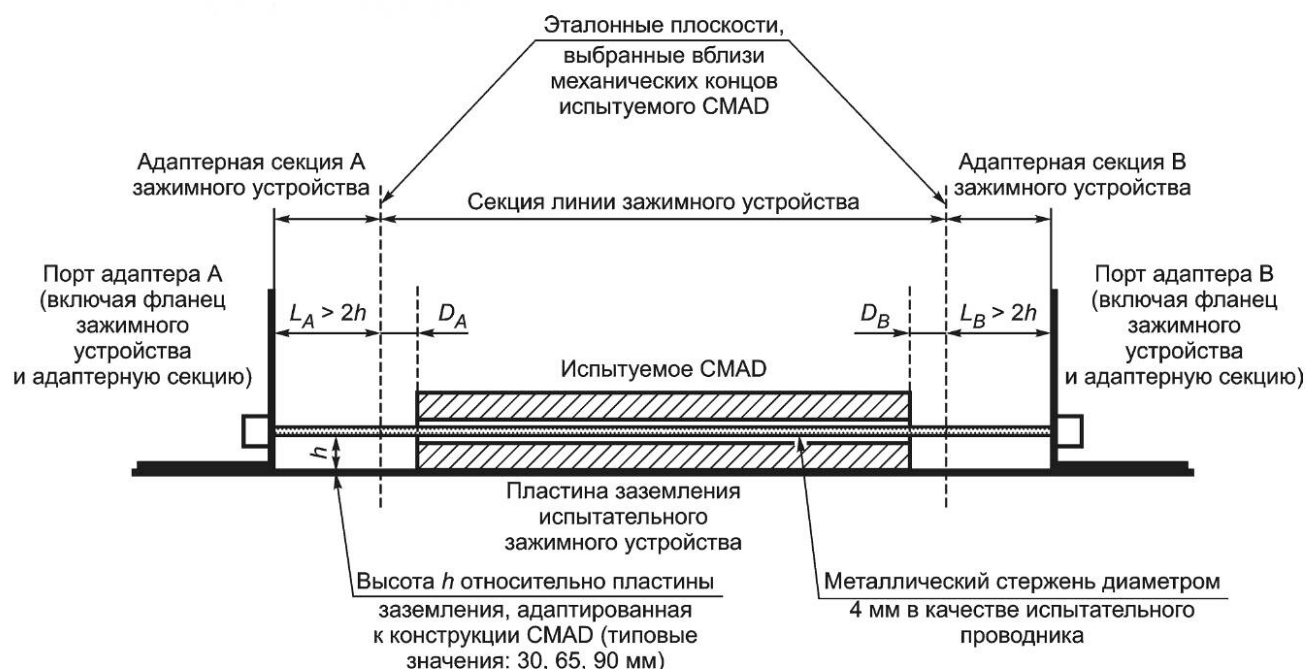
Рисунок 26 — Определение опорных плоскостей внутри испытательного зажимного устройства
