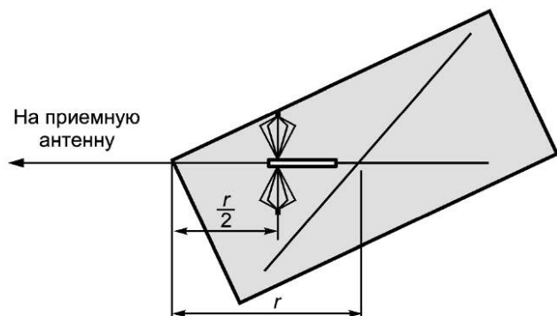
Рисунок 19 — Позиция антенны относительно края стола над прямоугольным установочным столом (вид сверху)
