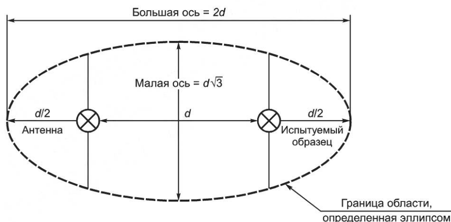
Рисунок 5 — Свободная от препятствий зона испытательной площадки с поворотным столом
