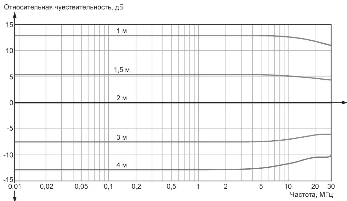
Рисунок С.10 — Чувствительность S_D LLA с диаметром D относительно LLA с диаметром 2 м
