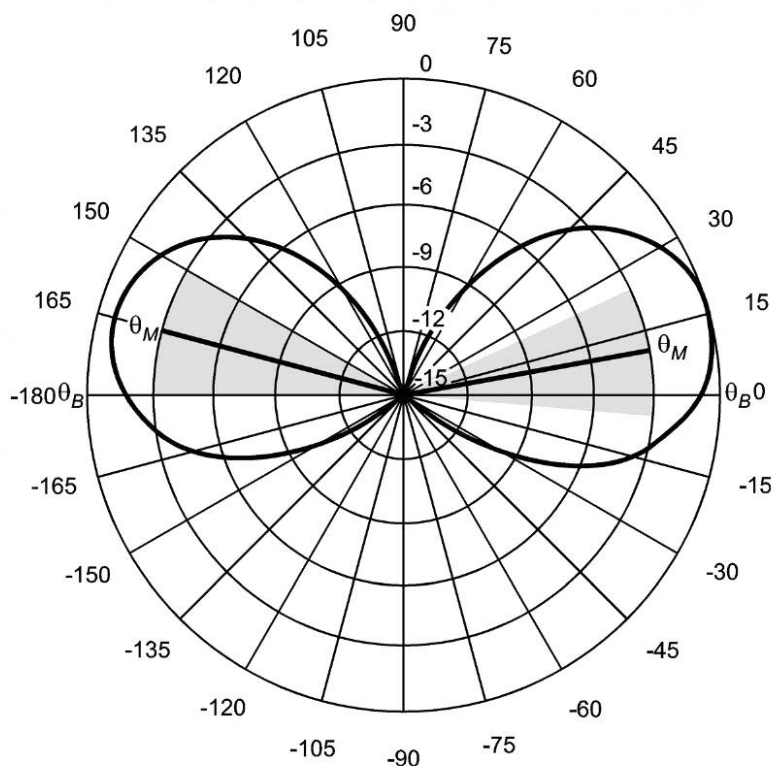
Рисунок 21 — Пример диаграммы направленности передающей антенны в плоскости E (только для информации)
