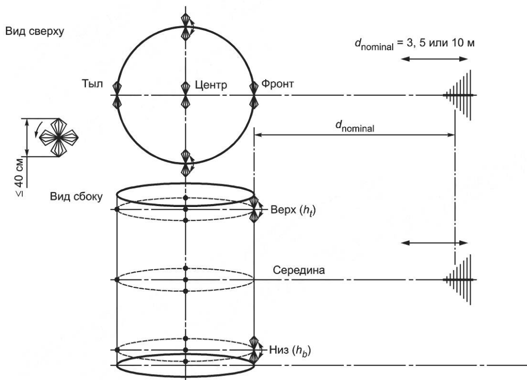
Рисунок 15 — Измерительные позиции при валидации площадки FAR
