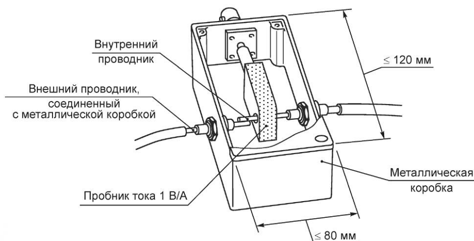
Рисунок С.5 — Конструкция металлической коробки с пробником тока
