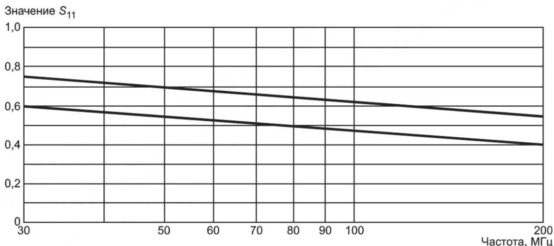
Рисунок 28 — Пределы для значения S_{11} , измеренного в соответствии с 8.1—8.3
