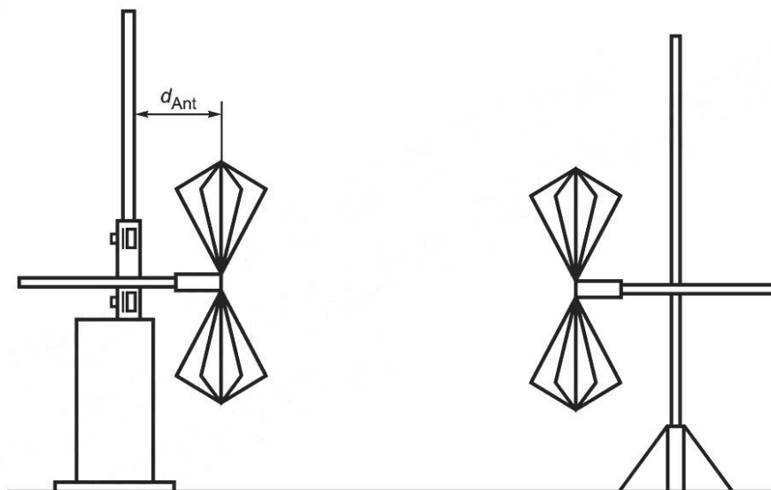
Рисунок 10 — Пример исследования влияния антенной мачты на A_{APR}
