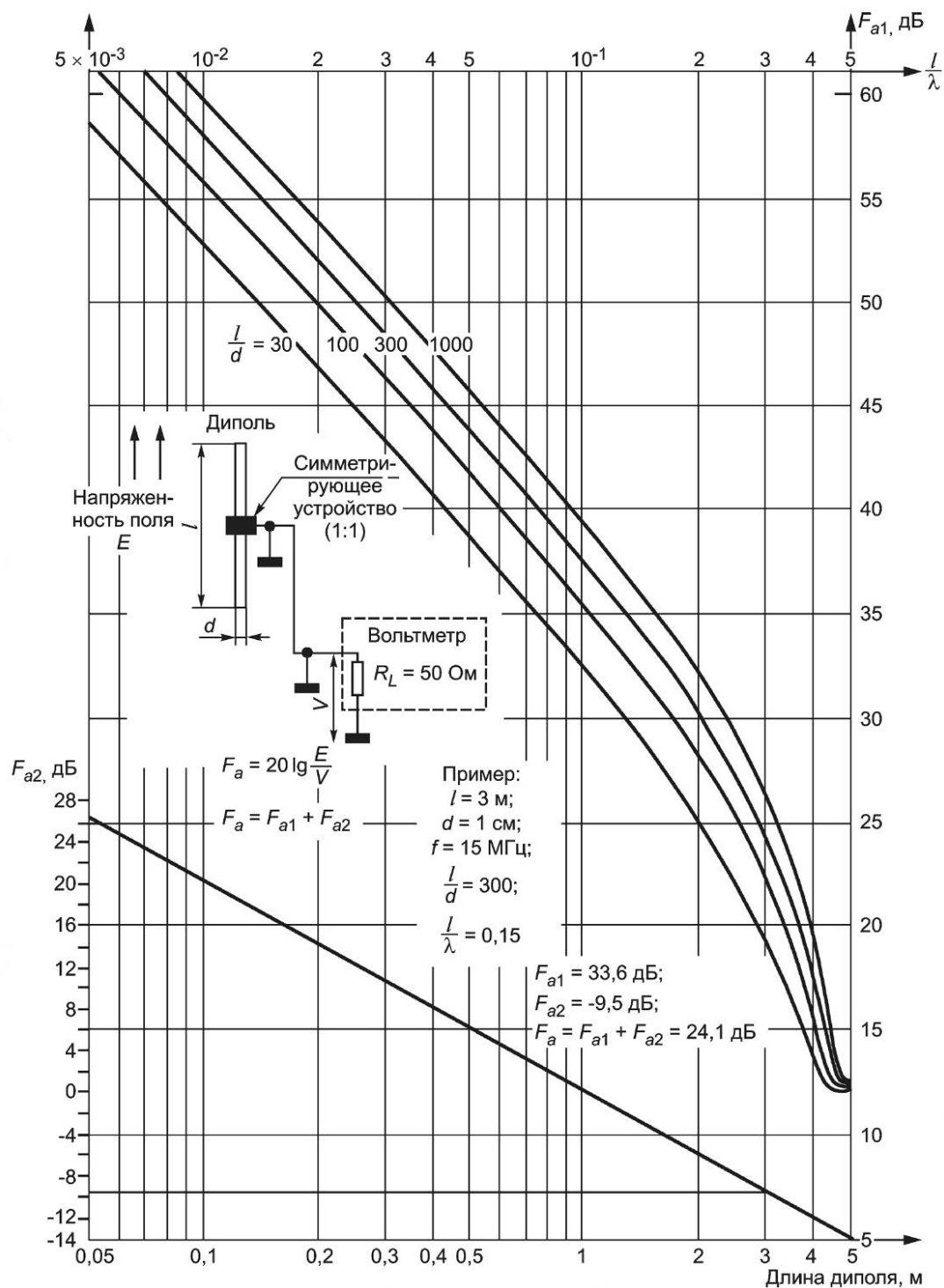
Рисунок А.1 — Коэффициенты калибровки антенны в виде короткого диполя при R_L = 50 \text{ Ом}
