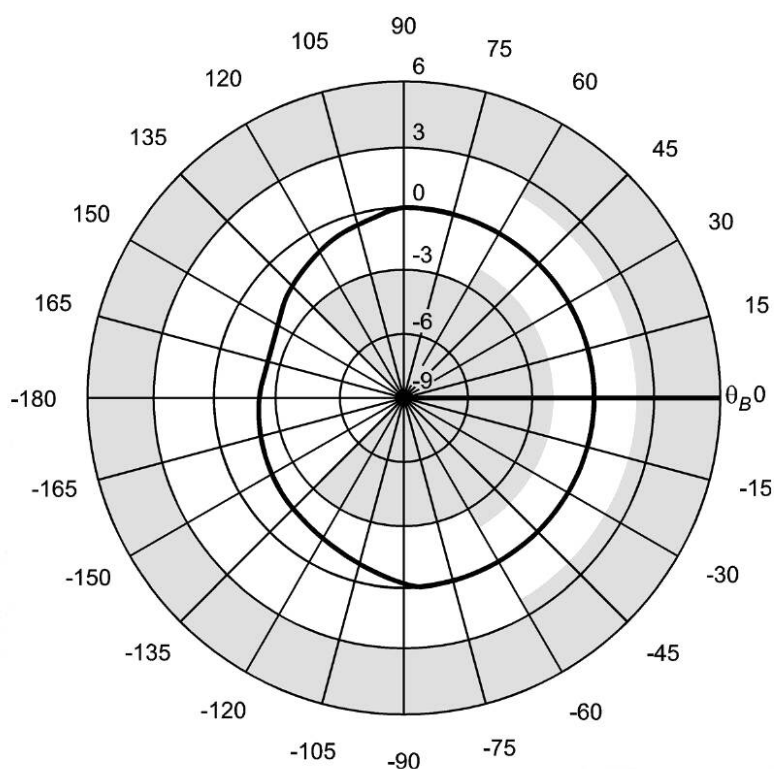
Рисунок 22a — Диаграмма направленности передающей антенны в плоскости H — от 1 до 6 ГГц
