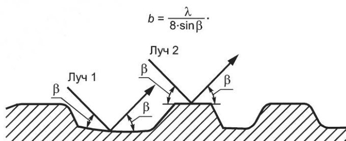
Рисунок D.1 — Критерий Релея для определения шероховатости поверхности пластины заземления
