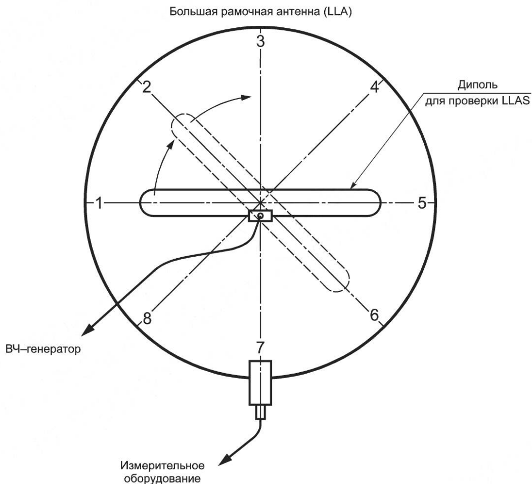
Рисунок С.7 — Восемь позиций дипольной антенны, используемой для проверки LLAS, во время валидации LLA
