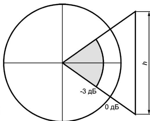
Рисунок 4 — Определение максимальной используемой высоты EUT с помощью ширины луча половинной мощности
