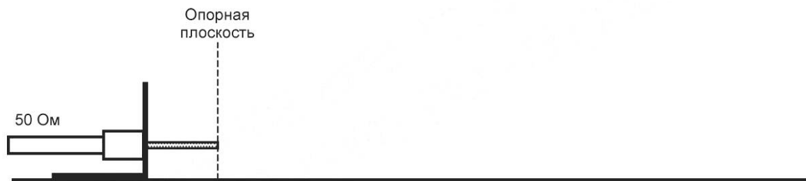
Рисунок 27а — Конфигурация при калибровочном измерении «отражение, порт А»
