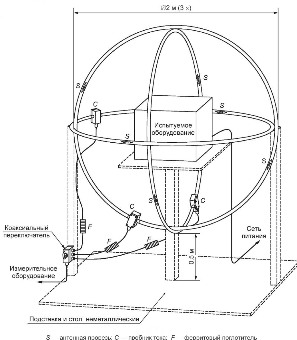
Рисунок С.1 — LLAS, состоящая из трех взаимно перпендикулярных больших рамочных антенн
