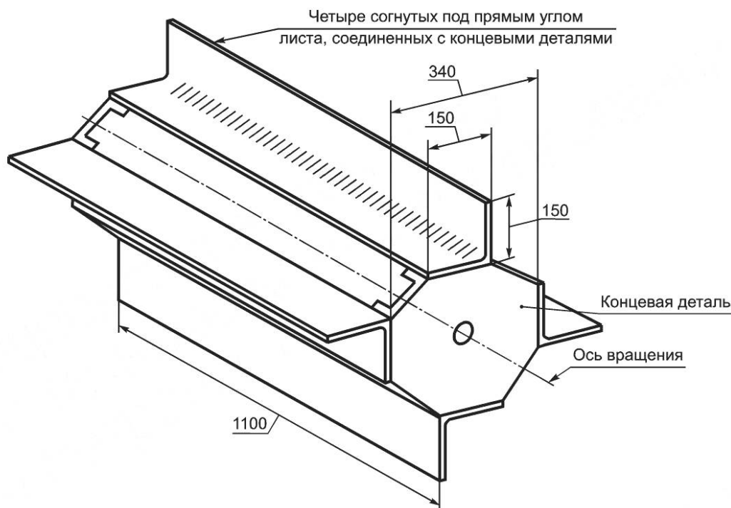
Рисунок 32 — Пример типичной лопаточной мешалки
