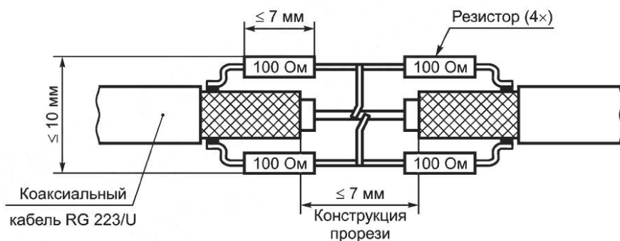
Рисунок С.3 — Конструкция прорези в LLA
