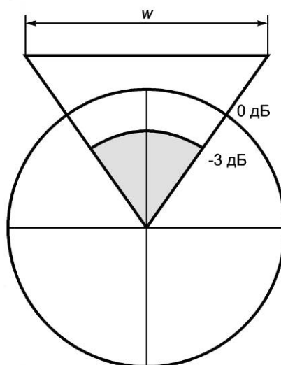
Рисунок 3 — Определение максимальной используемой ширины EUT с помощью ширины луча половинной мощности
