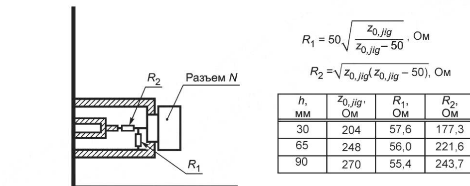
Рисунок 31 — Пример согласующего адаптера с резистивной схемой согласования
