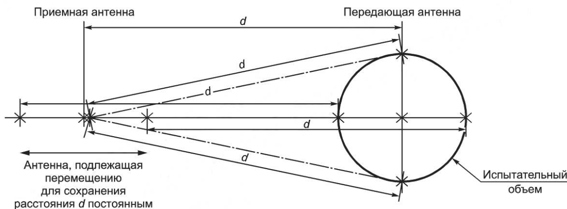
Рисунок 11 — Типичные позиции антенн для OATS с защитой от непогоды или SAC. Измерения параметров валидации при вертикальной поляризации
