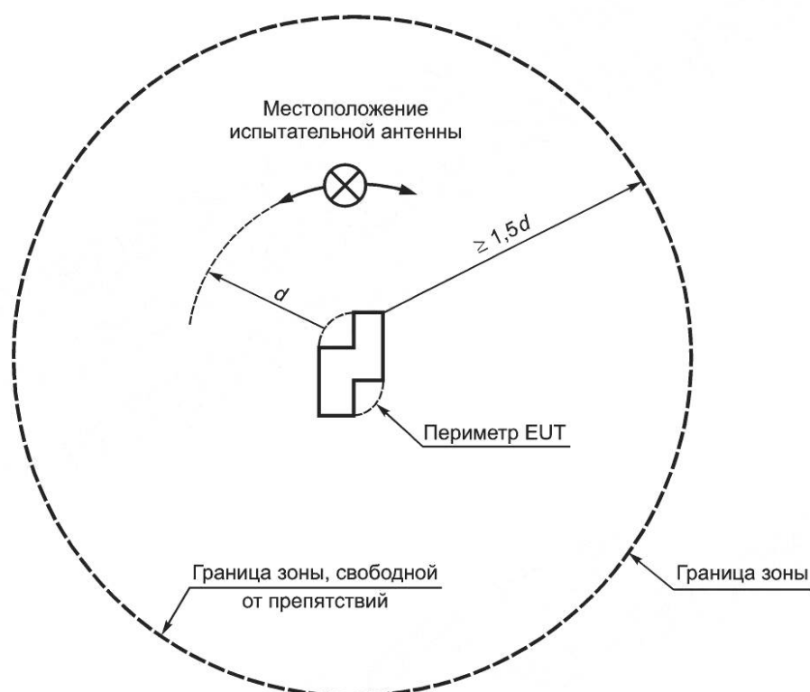
Рисунок 6 — Зона, свободная от препятствий, со стационарным испытуемым оборудованием
