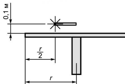
Рисунок 20 — Позиция антенны над установочным столом (вид сбоку)
