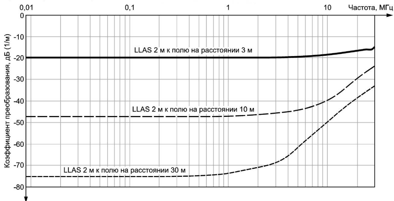
Рисунок С.11 — Коэффициент преобразования C_{dA} [для приведения к дБ (мкА/м)] для трех стандартных измерительных расстояний d
