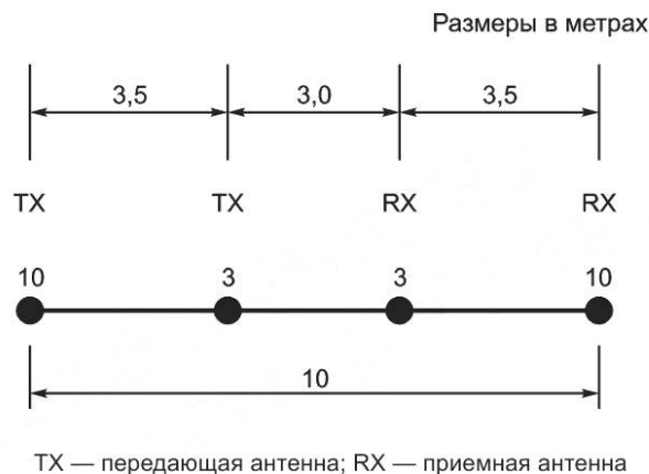
Рисунок 7 — Расположение испытательных точек при испытательных расстояниях 3 и 10 м
