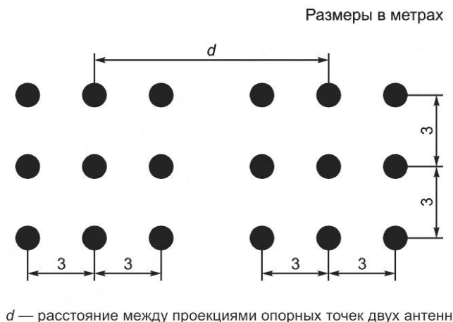
Рисунок 8 — Позиции парных испытательных точек при всех испытательных расстояниях
