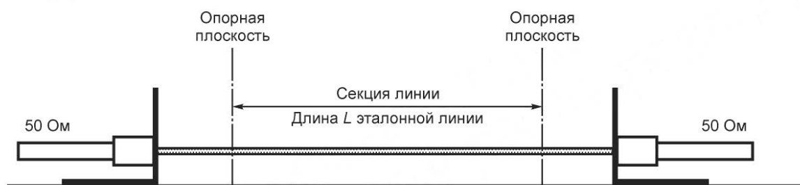
Рисунок 27d — Конфигурация при калибровочном измерении «линия»
