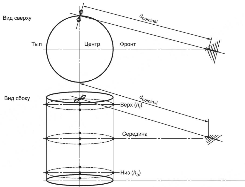
Рисунок 16 — Пример одной измерительной позиции и наклона антенны при валидации площадки FAR
