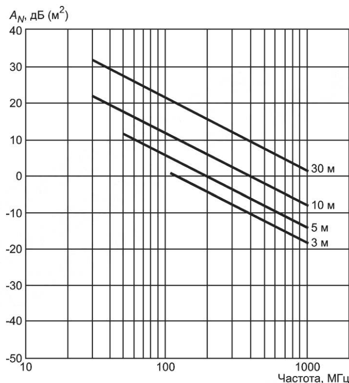
Рисунок 18 — Теоретическое NSA в условиях свободного пространства как функция частоты при разных измерительных расстояниях [см. уравнение (16)]
