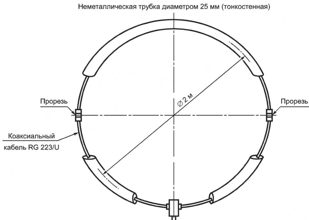
Рисунок С.2 — LLA с двумя прорезями на противоположных сторонах, расположенными симметрично относительно пробника тока С
