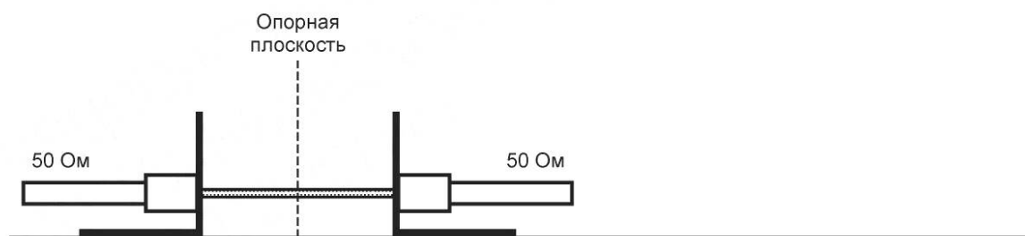
Рисунок 27c — Конфигурация при калибровочном измерении «насквозь»
