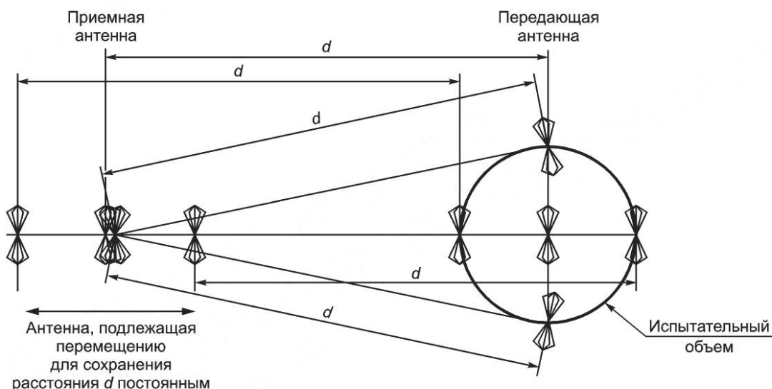
Рисунок 12 — Типичные позиции антенн для OATS с защитой от непогоды или SAC. Измерения параметров валидации при горизонтальной поляризации
