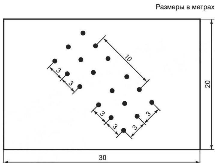
Рисунок 9 — Пример выбора парных испытательных точек при испытательном расстоянии 10 м
