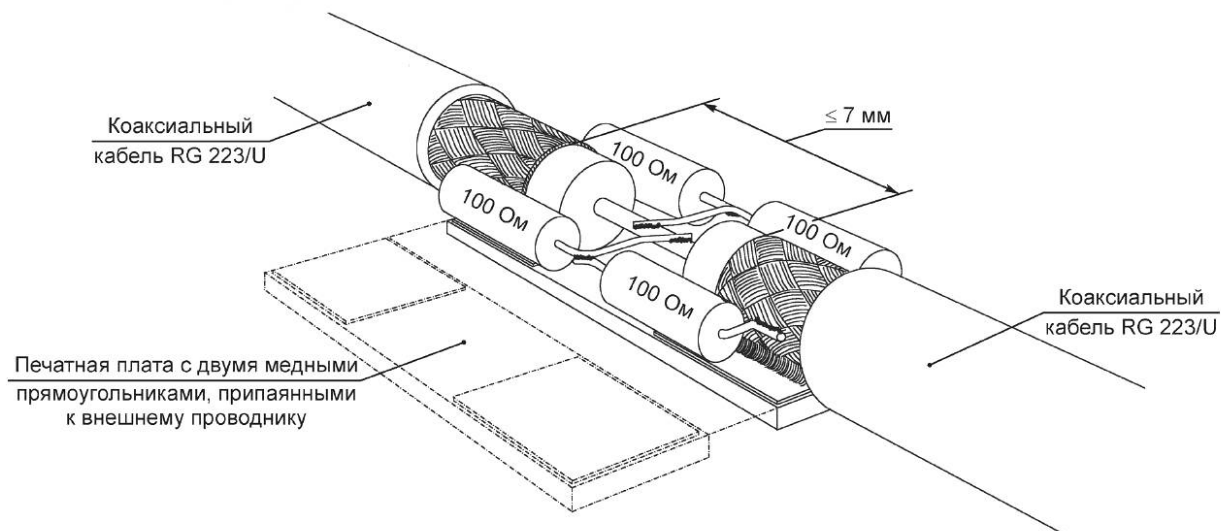
Рисунок С.4 — Пример конструкции прорези LLA с использованием перемычки из материала печатной платы для обеспечения жесткой конструкции
