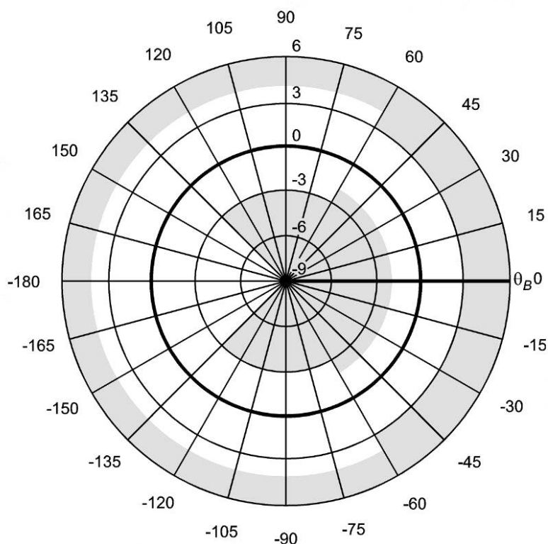
Рисунок 22b — Диаграмма направленности передающей антенны в плоскости H — от 6 до 18 ГГц
