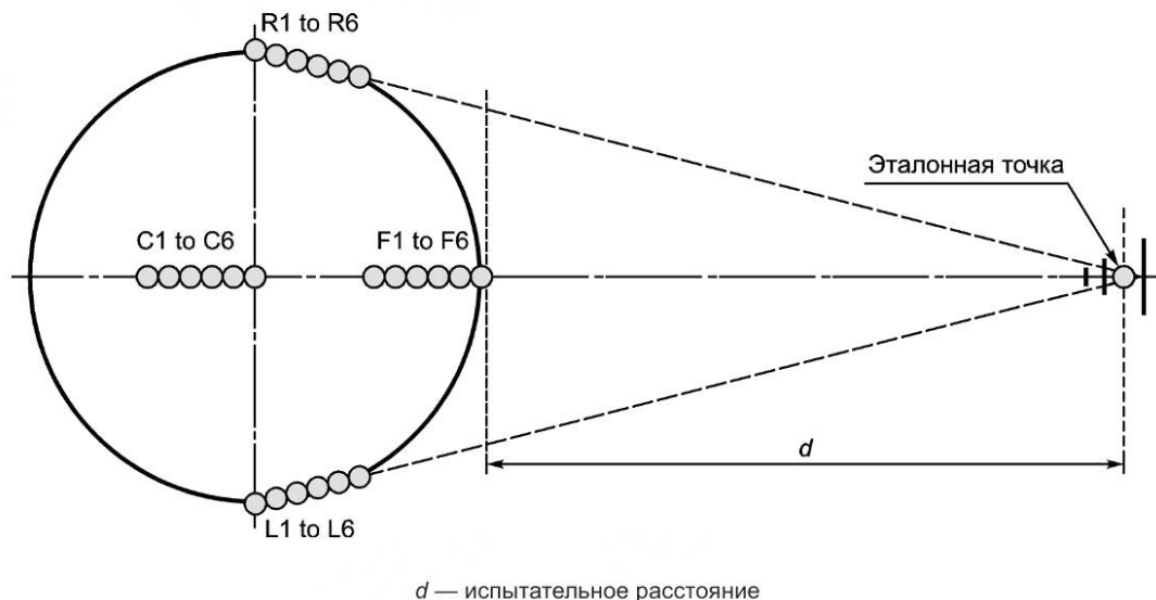
Рисунок 23 — Позиции при измерении S_{VSWR} в горизонтальной плоскости (см. 7.5.2)
