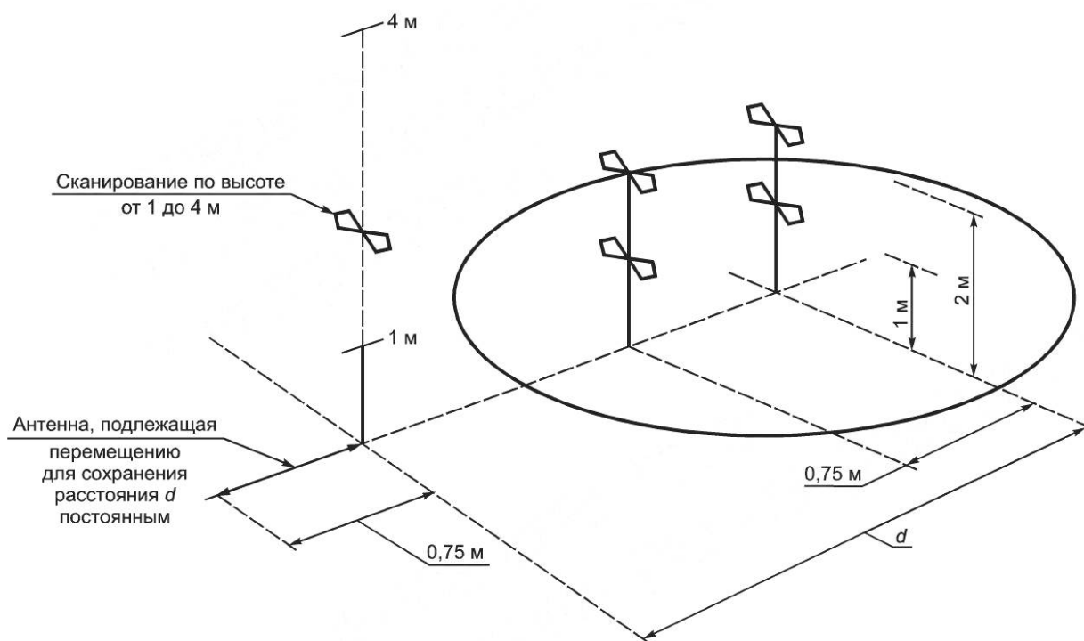
Рисунок 13 — Типичные позиции антенны для OATS с защитой от непогоды или SAC. Измерения параметров валидации при вертикальной поляризации для EUT небольшого размера
