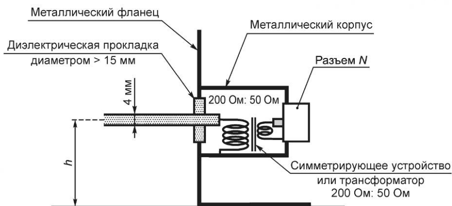
Рисунок 29 — Пример конструкции адаптера 50 Ом в вертикальном фланце зажимного устройства
