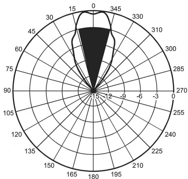
Рисунок 2 — Пример диаграммы направленности приемной антенны в плоскости E с ограничительной областью, заштрихованной для расстояния 3 м и размера EUT 2 м
