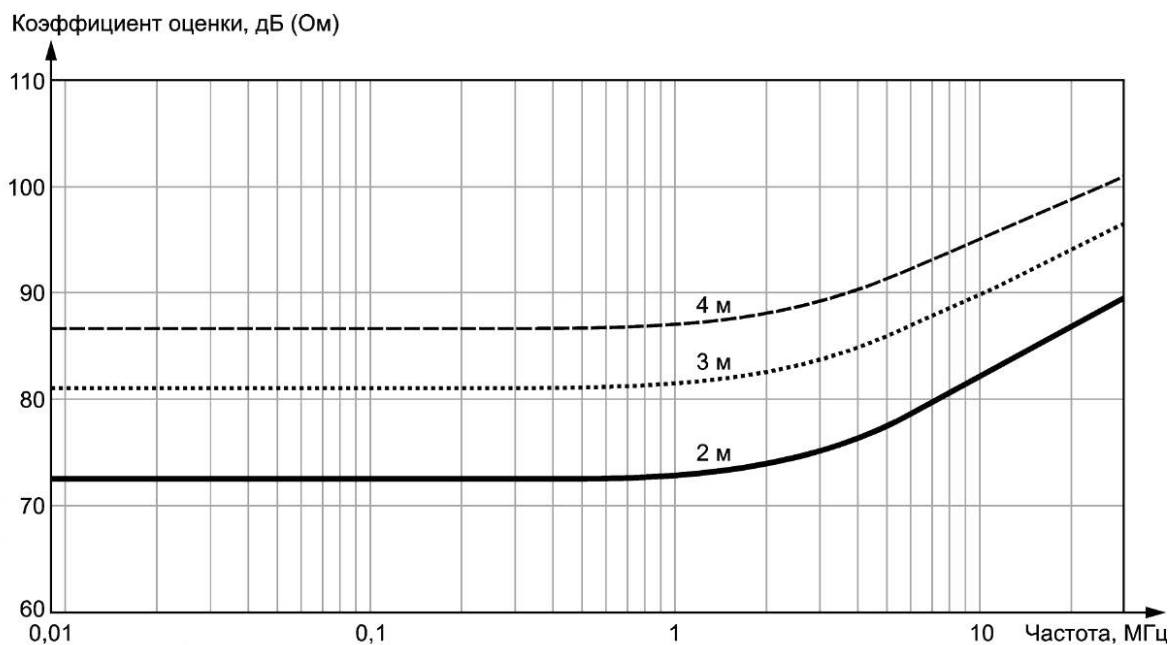
Рисунок С.8 — Эталонные коэффициенты оценки для рамочных антенн с диаметрами 2, 3 м и 4 м
