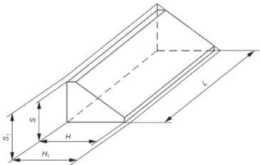
Рисунок 6 — Фасонное изделие
