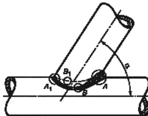
Рисунок 7 — Вырезка образцов для испытаний из таврового соединения
