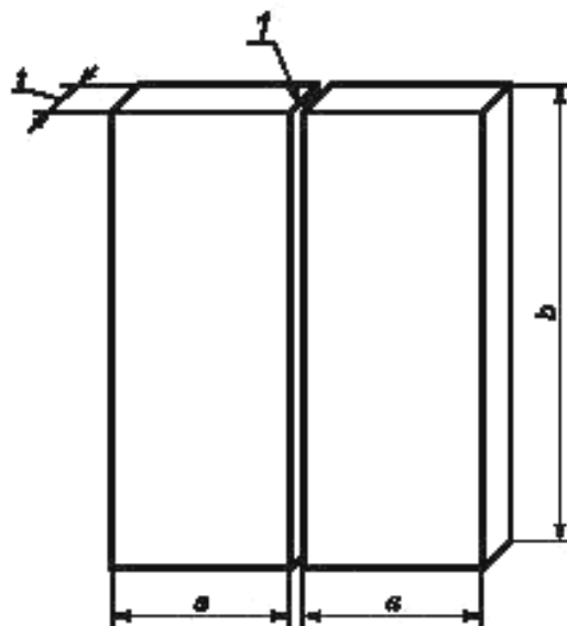
t — подготовка и сборка соединения, как описано в pWPS; a — минимальное значение 150 мм; b — минимальное значение 350 мм; f — толщина материала
