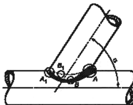
Рисунок 7 — Вырезка образцов для испытаний из таврового соединения
