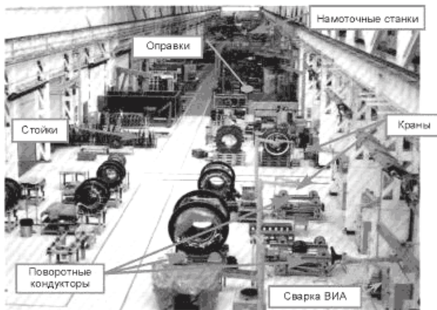
Рисунок В.2 — Пример сборочного цеха
