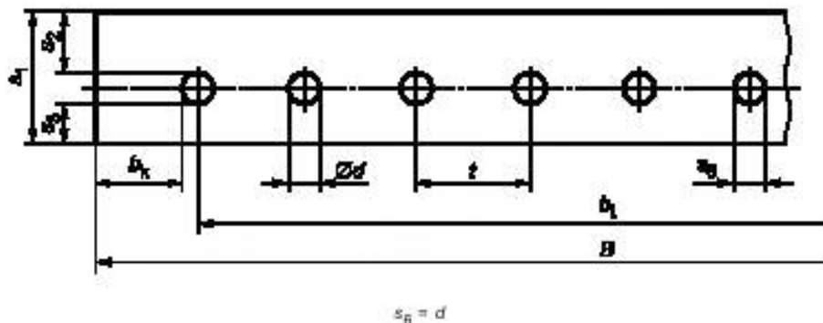
Рисунок 1 — Поперечное сечение ленты стандартного типа
