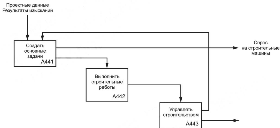
Рисунок Е.3 — Рабочий процесс на строительной площадке (IDEF0)
