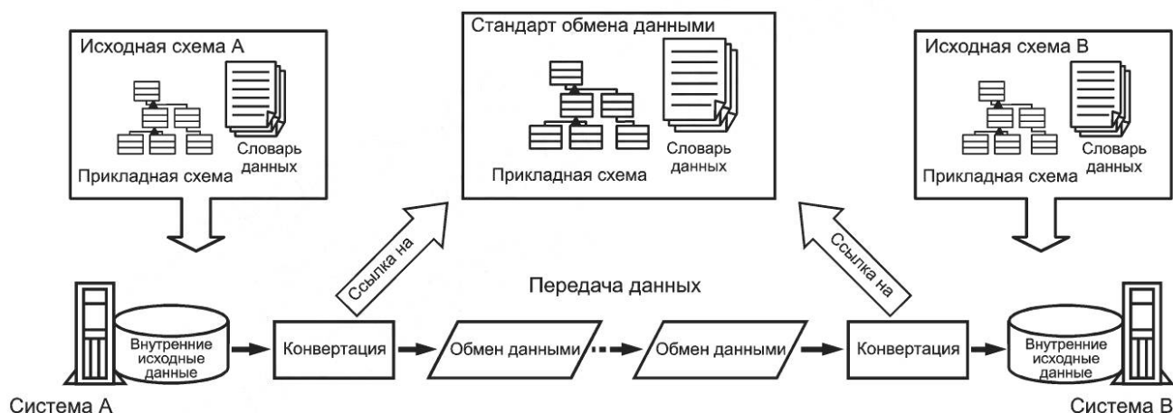
Рисунок 2 — Модель передачи данных
