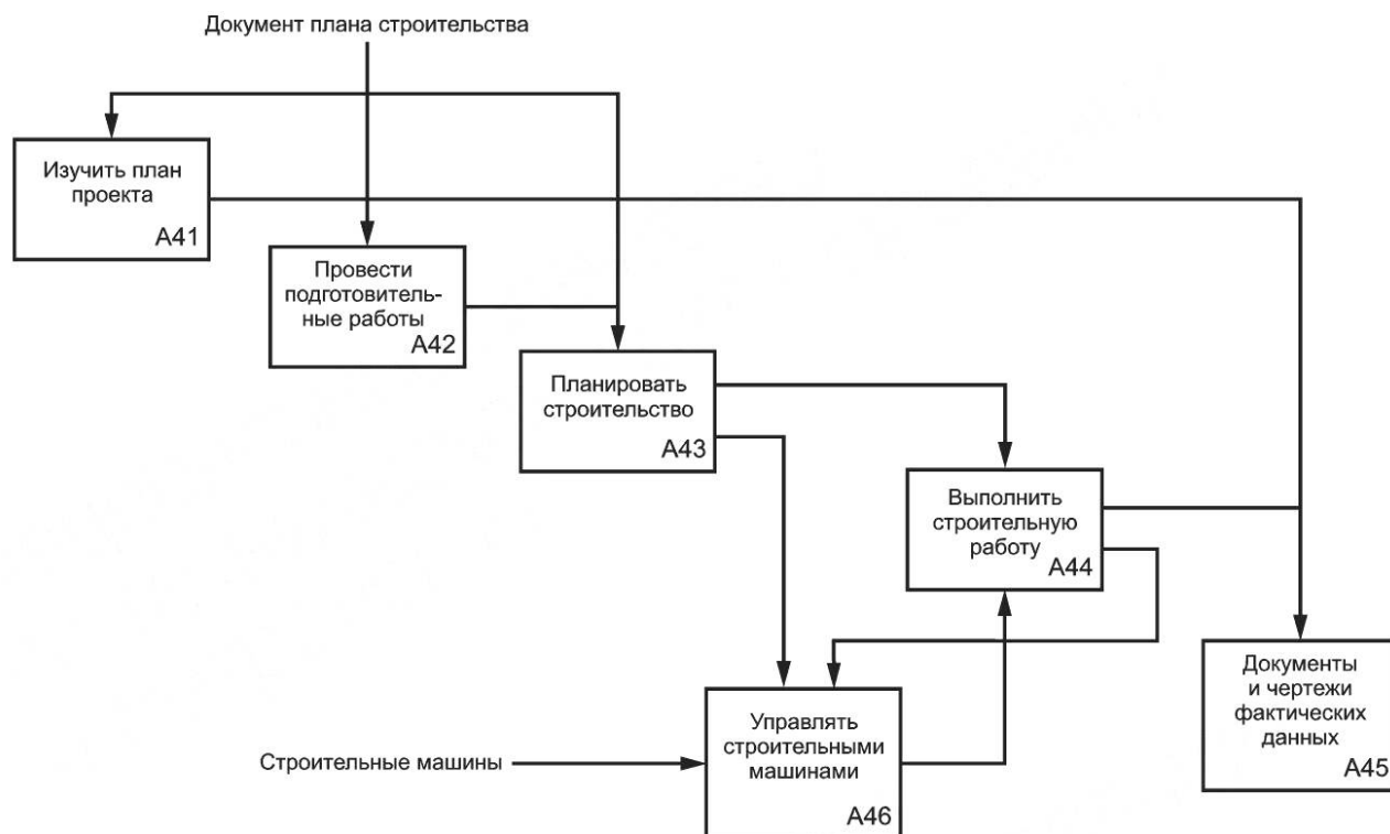
Рисунок Е.2 — Рабочий процесс этапа строительства (IDEF0)
