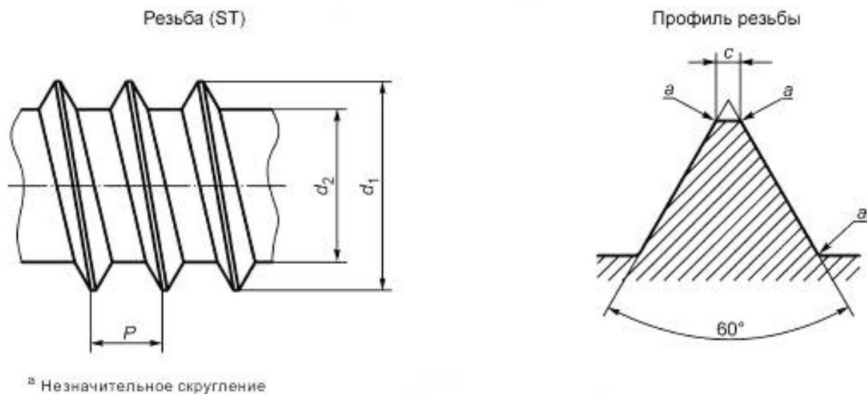
Рисунок 1 — Размеры резьбы
