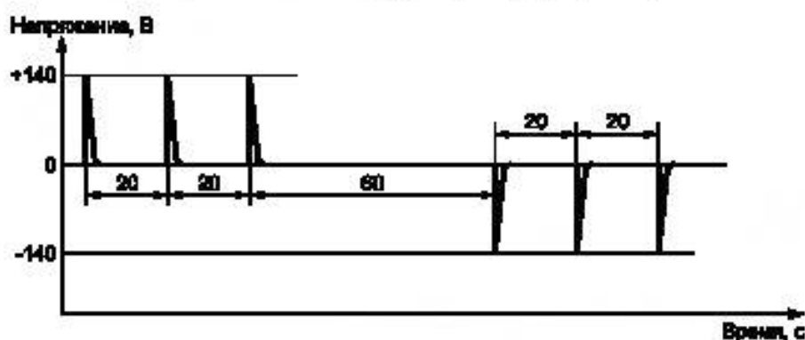
Рисунок 2 — Форма импульсов, используемых при дефибриляции
