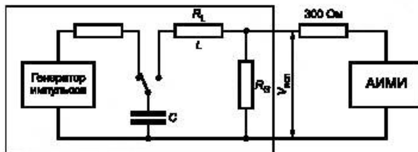
Рисунок 1 — RCL контур для оценки дефибриляции
