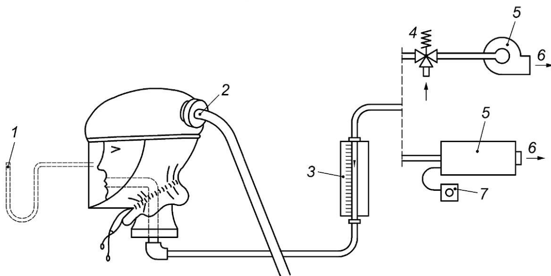
Рисунок 9 — Типовая установка для измерения расхода воздуха при использовании неплотно прилегающей лицевой части
