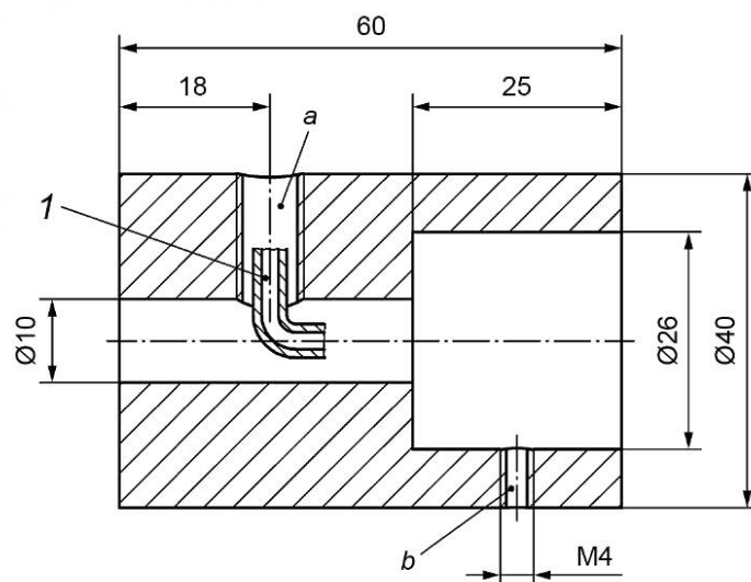
1 — внешний диаметр 4 мм, внутренний диаметр 2 мм; a — соединение контрольного устройства; b — местоположение зажимного винта для закрепления на сопле во время регулировки давления
