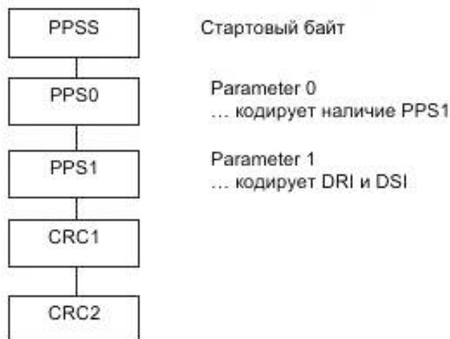
Рисунок 9 – Запрос выбора протокола и параметров
