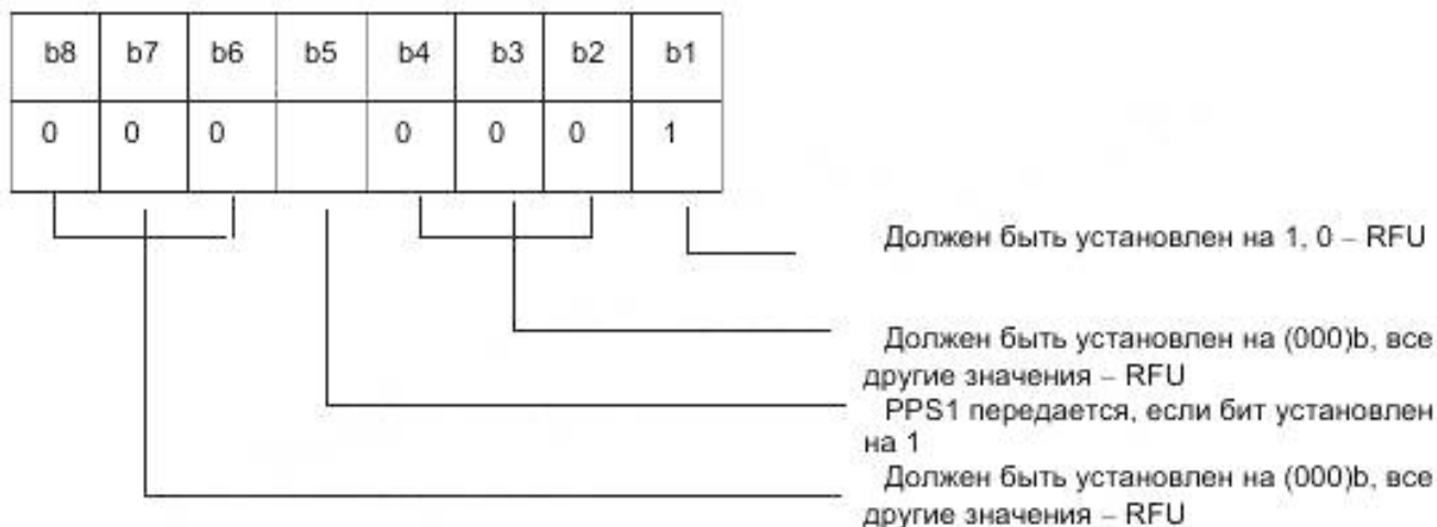
Рисунок 11 – Кодирование PPS0
