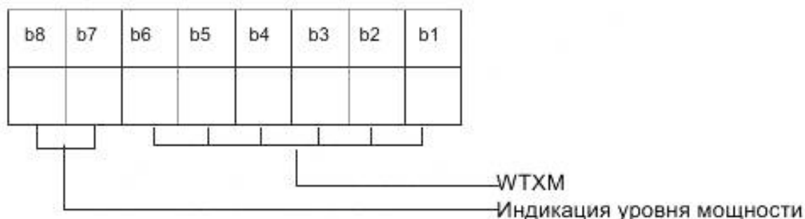
Рисунок 20 – Кодирование INF при запросе S(WTX)
