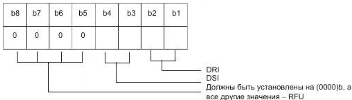
Рисунок 12 – Кодирование PPS1
