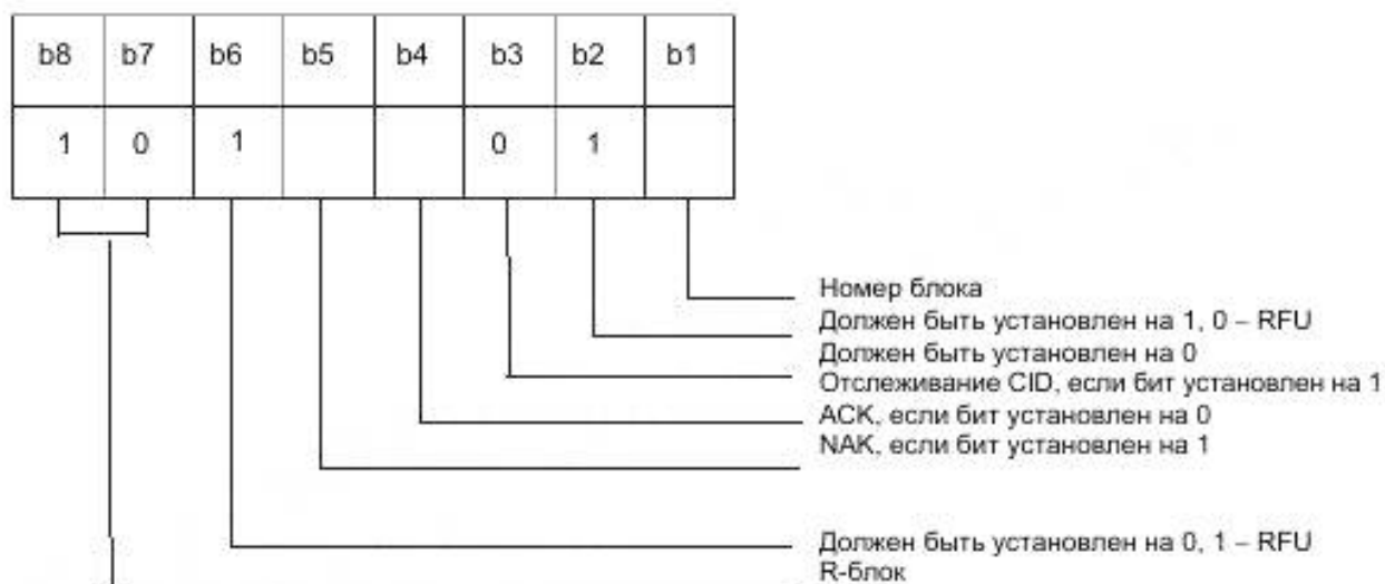
Рисунок 16 – Кодирование R-блока PCB
