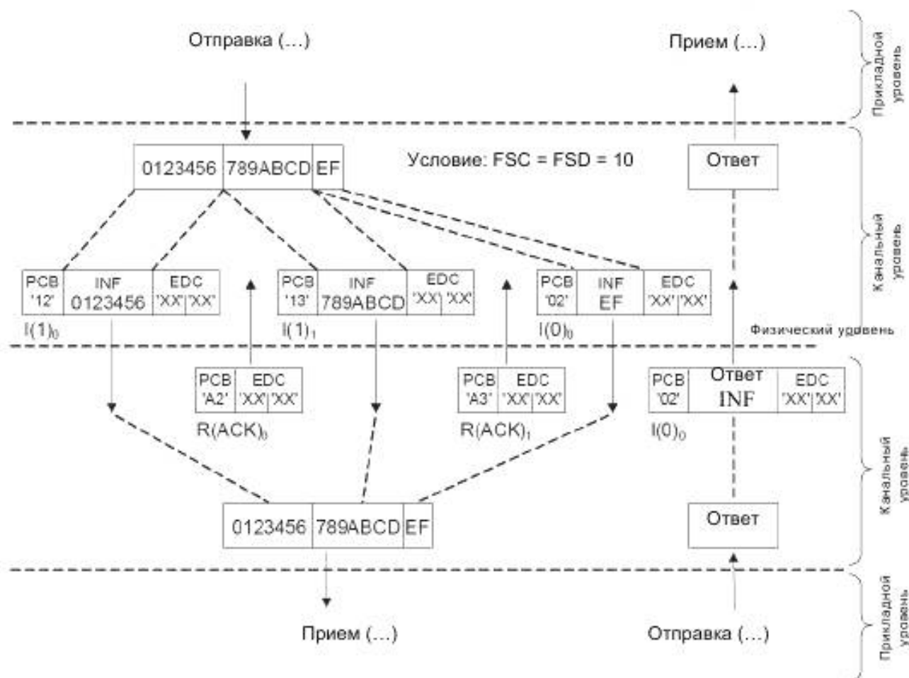
Рисунок 22 – Сцепление
