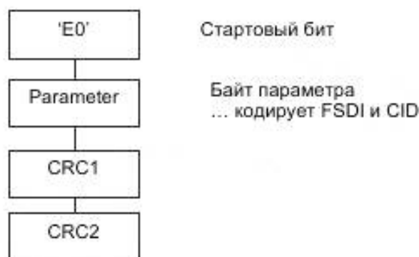
Рисунок 2 – Запрос для Ответа на Выбор
