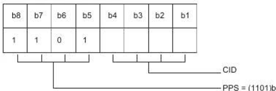
Рисунок 10 – Кодирование PPSS
