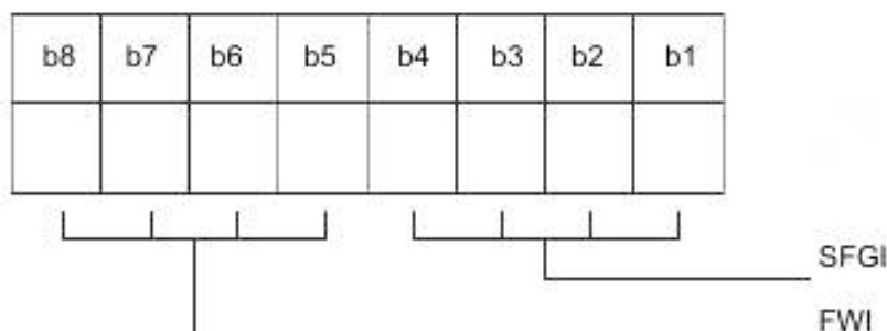
Рисунок 7 – Кодирование байта интерфейса TB(1)
