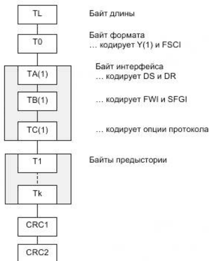
Рисунок 4 – Структура ATS
