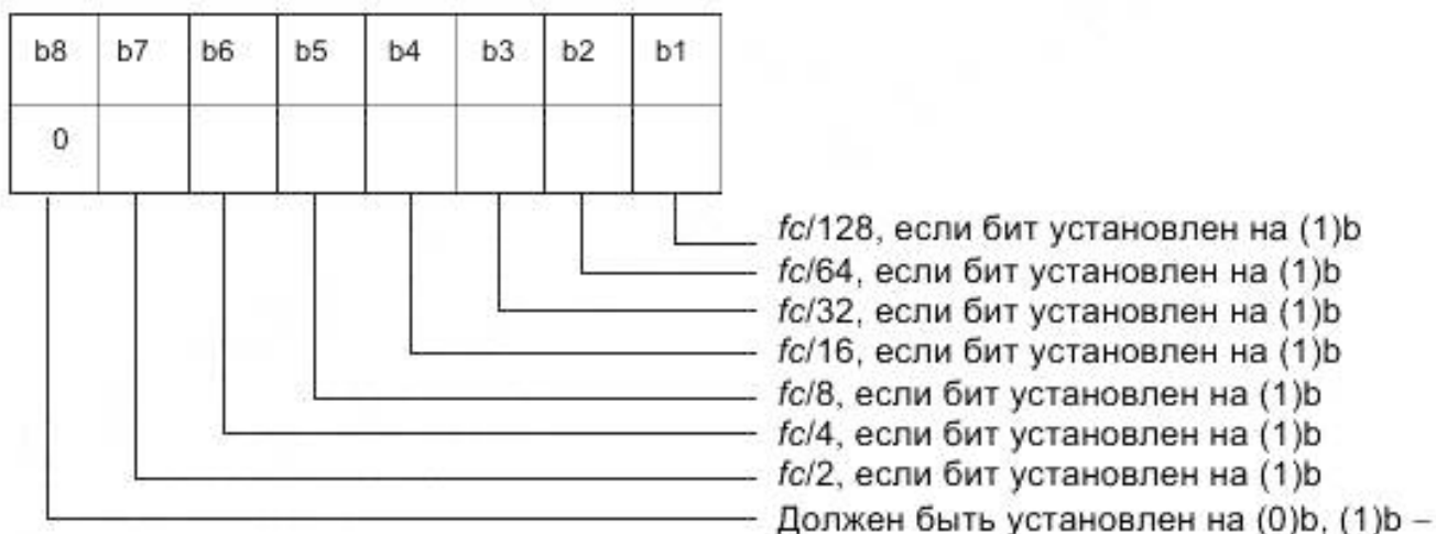
Рисунок 23 – Кодирование скоростей передачи
