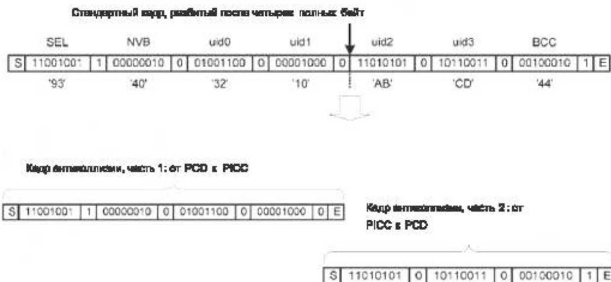
Рисунок 5 – Организация бит и передача бит-ориентированного кадра антиколлизии, случай FULL BYTE
