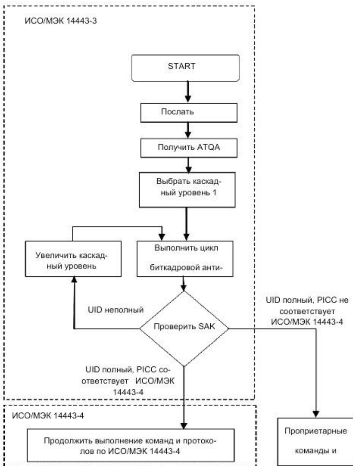
Рисунок 9 – Блок-схема инициализации и антиколлизии для PCD
