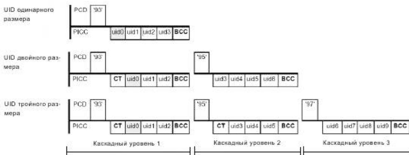
Рисунок 12 – Использование каскадных уровней
