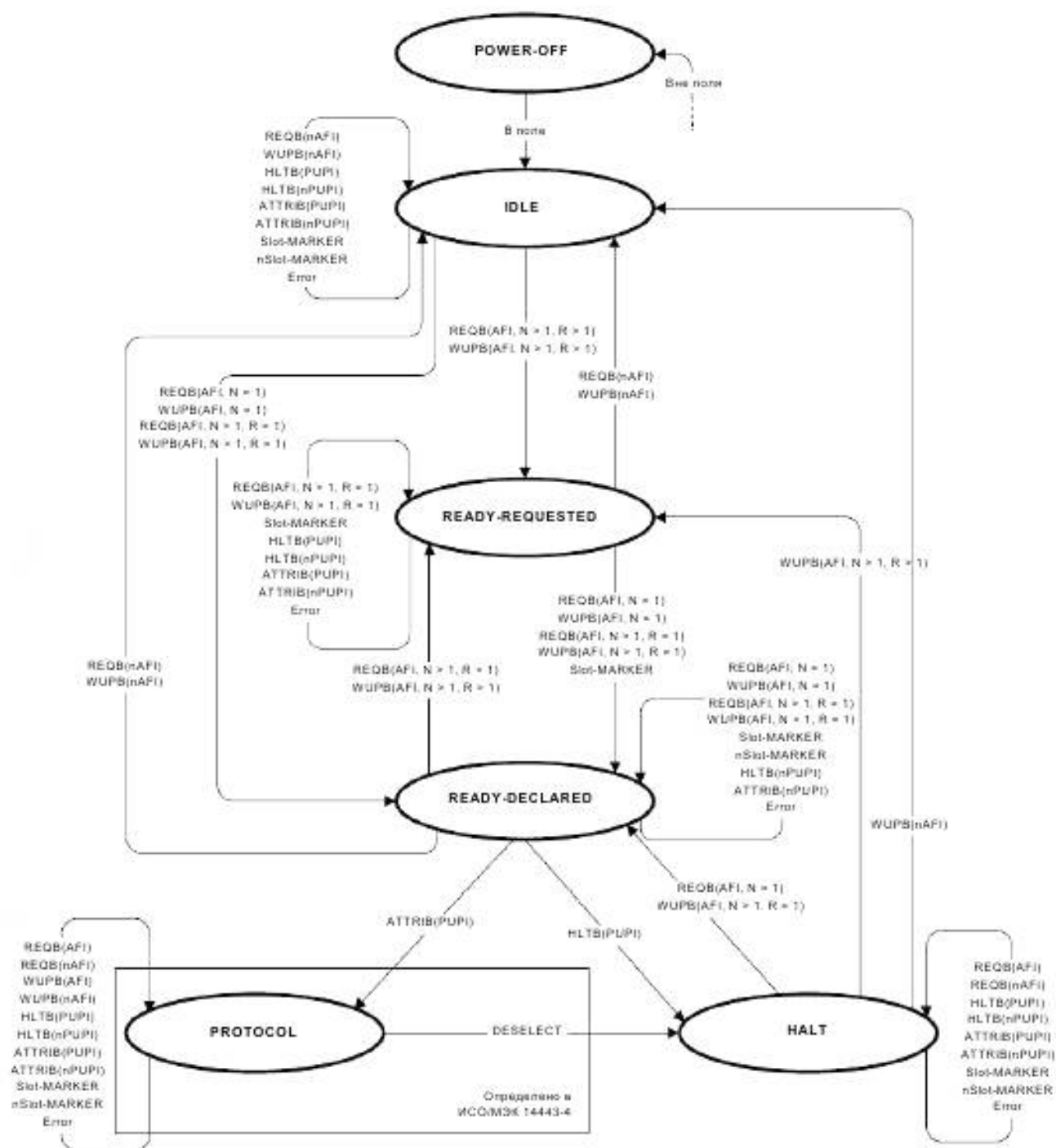
Рисунок 19 – Диаграмма состояний PICC типа В
