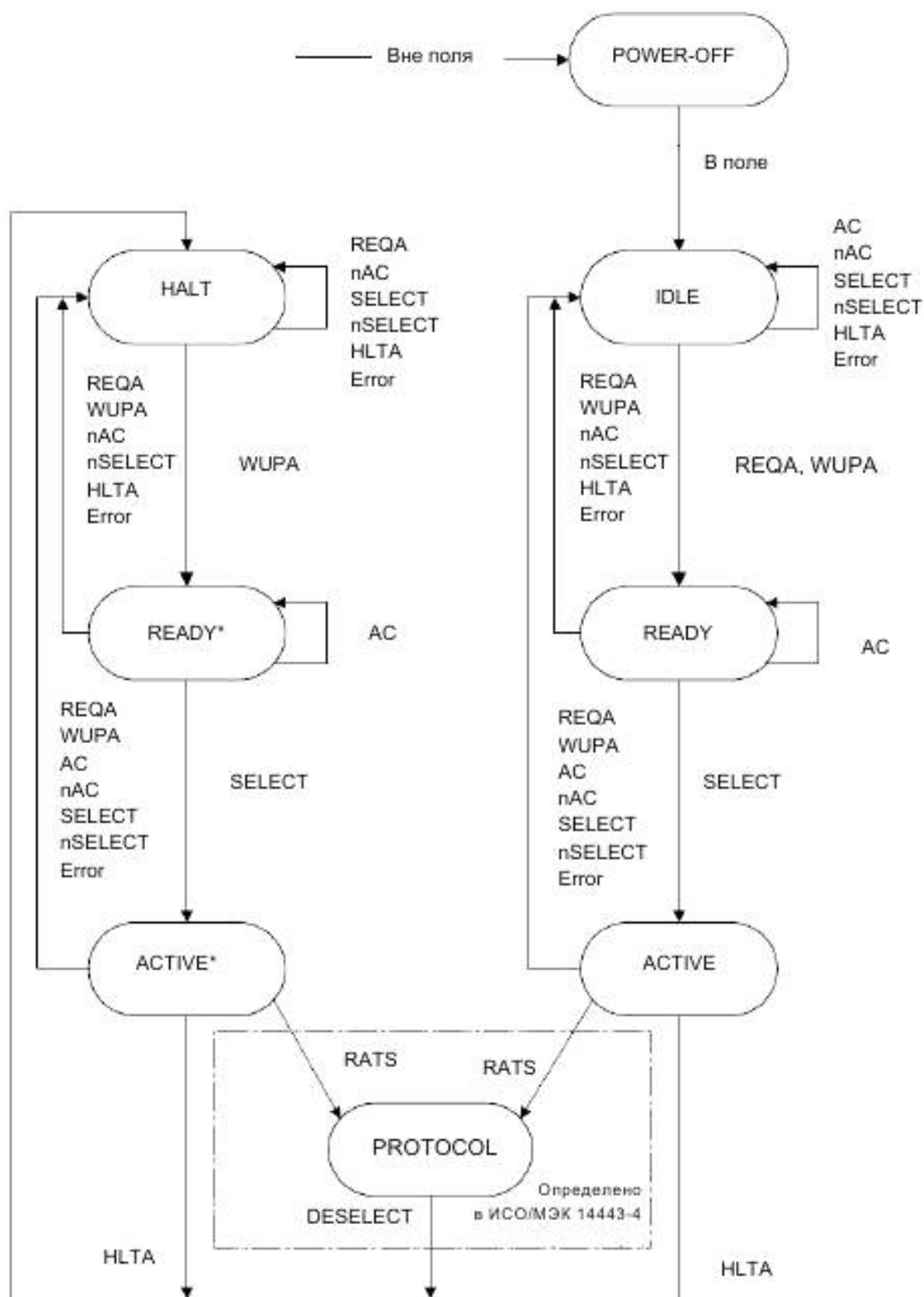
Рисунок 7 – Диаграмма состояний PICC типа A
