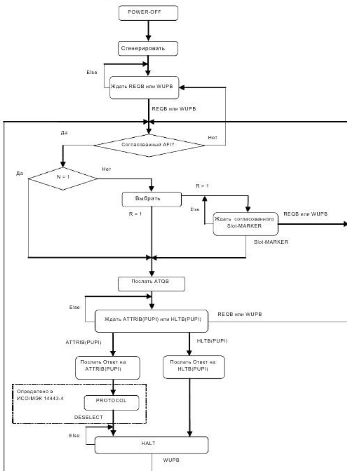
Рисунок 20 – Блок-схема инициализации и антиколлизии PICC
