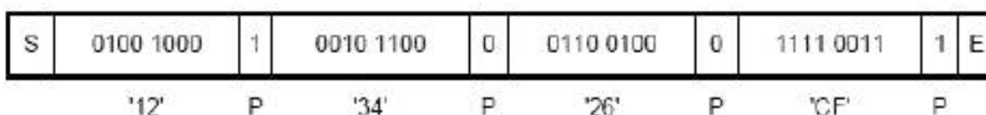
Рисунок В.2 – Пример 2 для кодирования CRC_A
