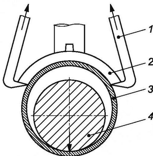
Рисунок 1 — Схема испытания для оборудования типа A1
