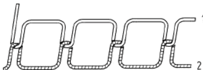
1 – игловая нить; 2 – шпулечная нить
