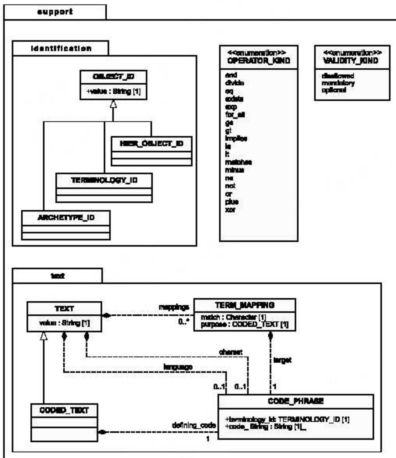
Рисунок 12 — Пакет support
