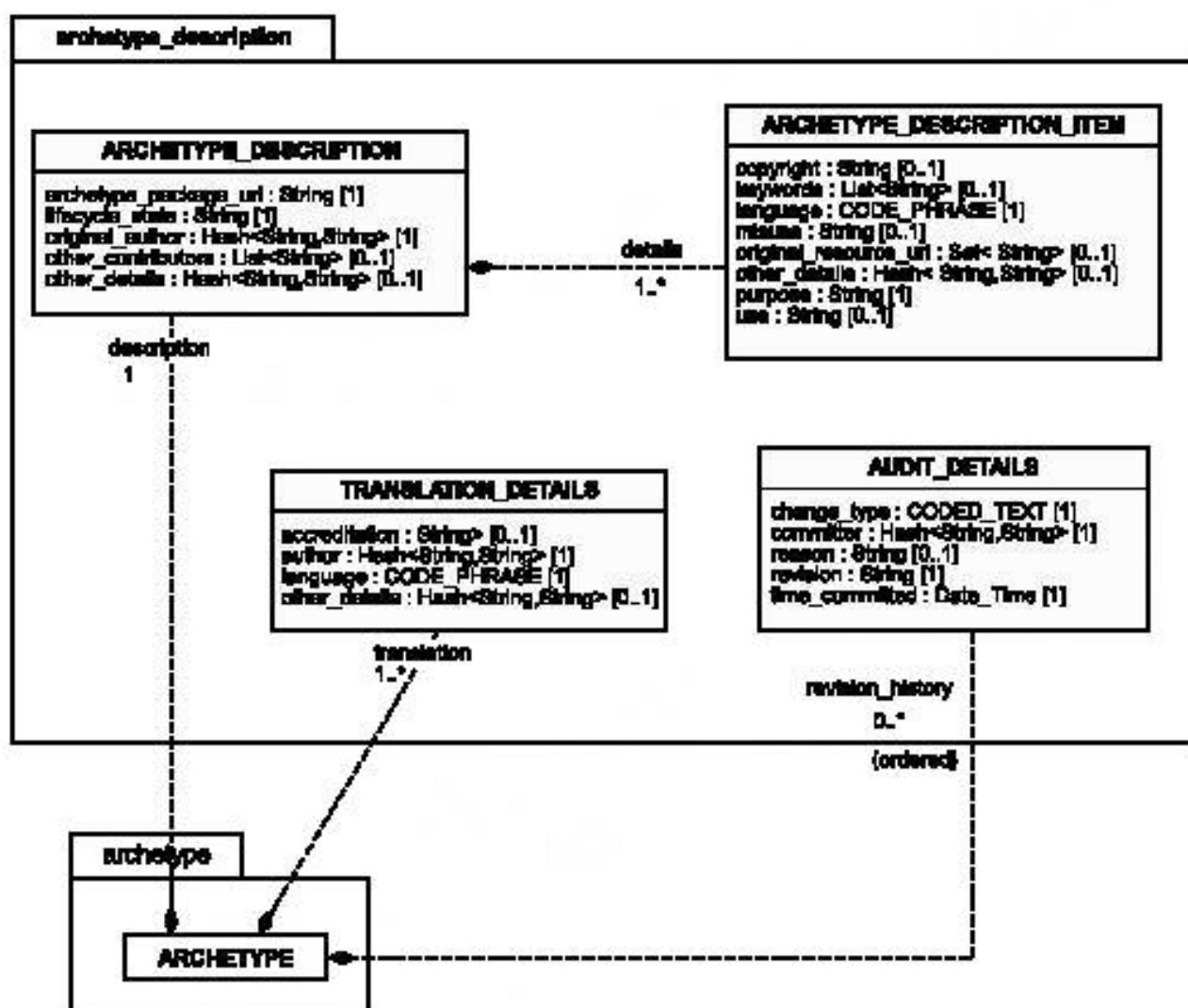
Рисунок 6 — Пакет archetype_description
