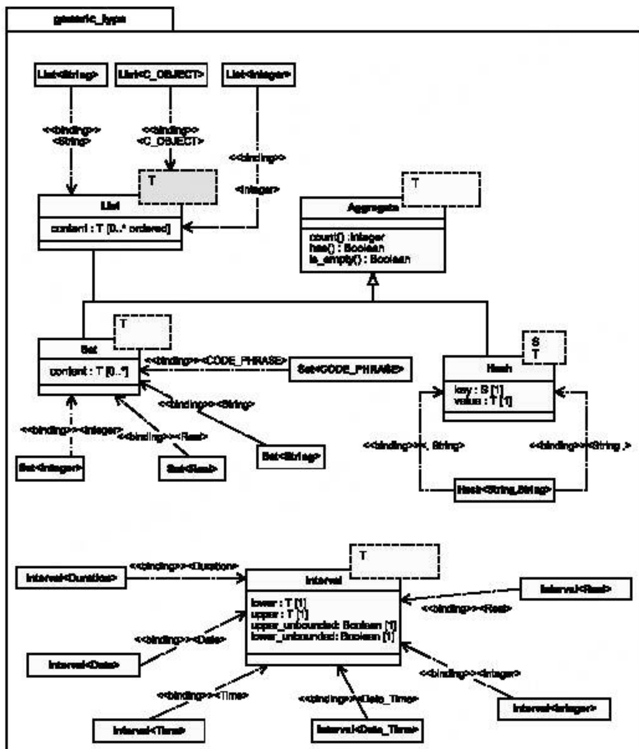
Рисунок 13 — Пакет generic_types
