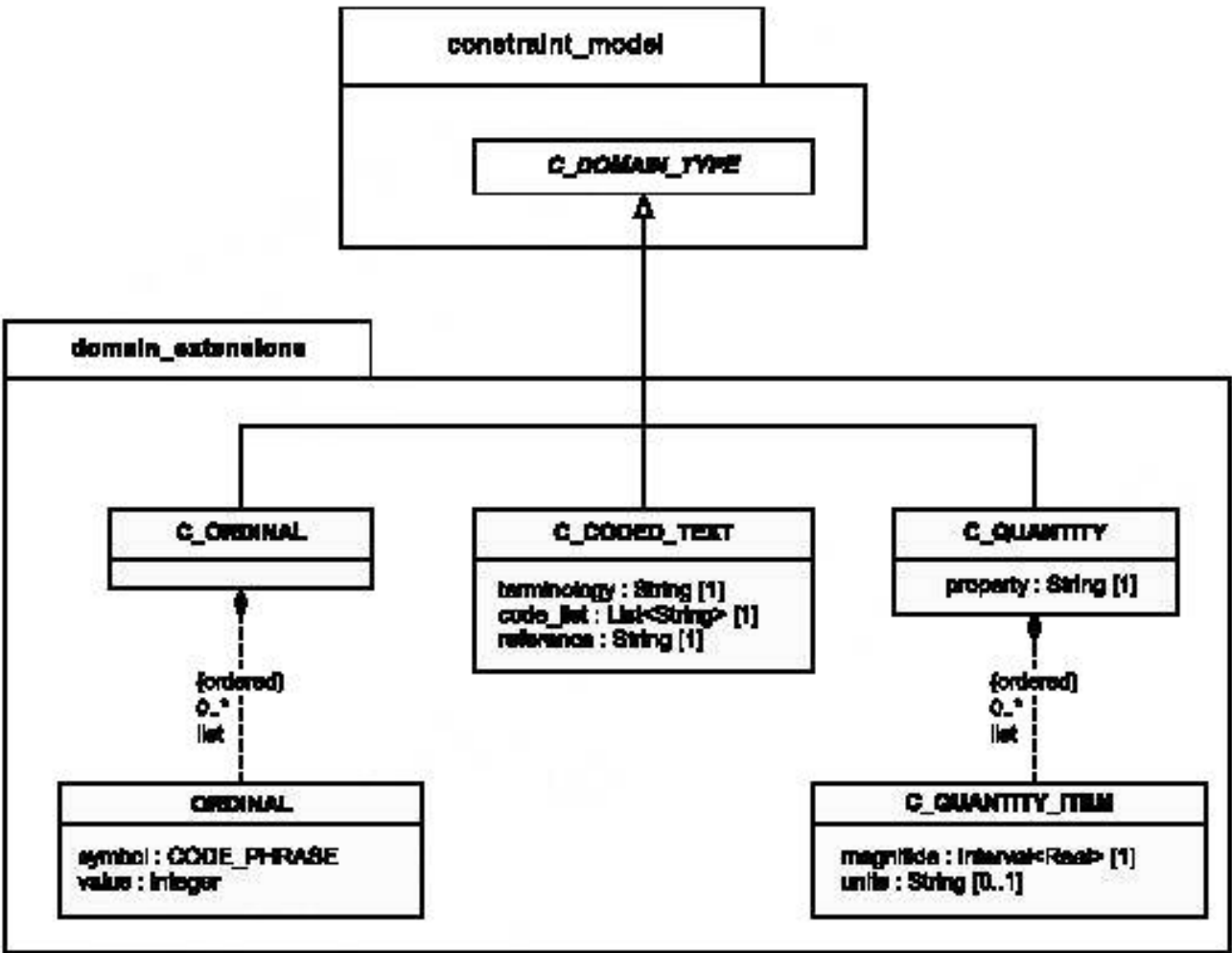
Рисунок 11 — Пакет domain_extensions
