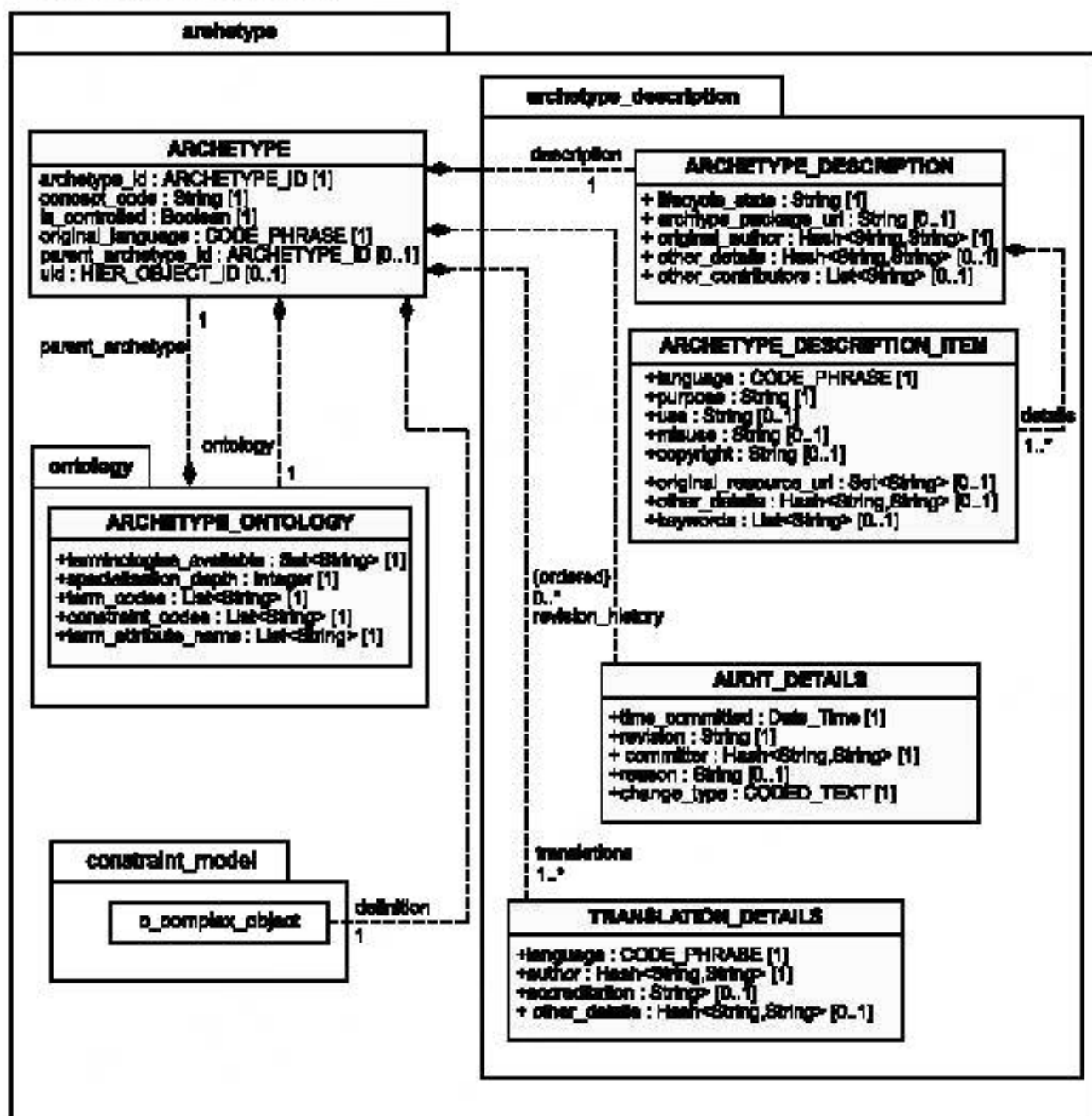
Рисунок 5 — Пакет archetype
