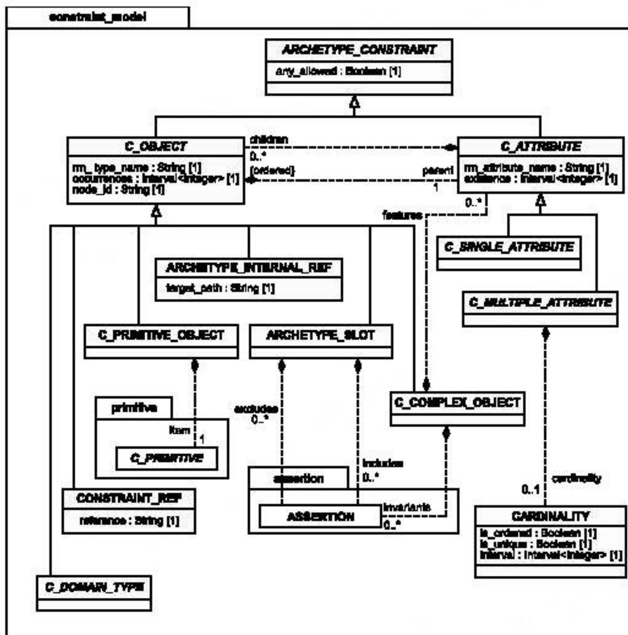
Рисунок 7 — Пакет constraint_model
