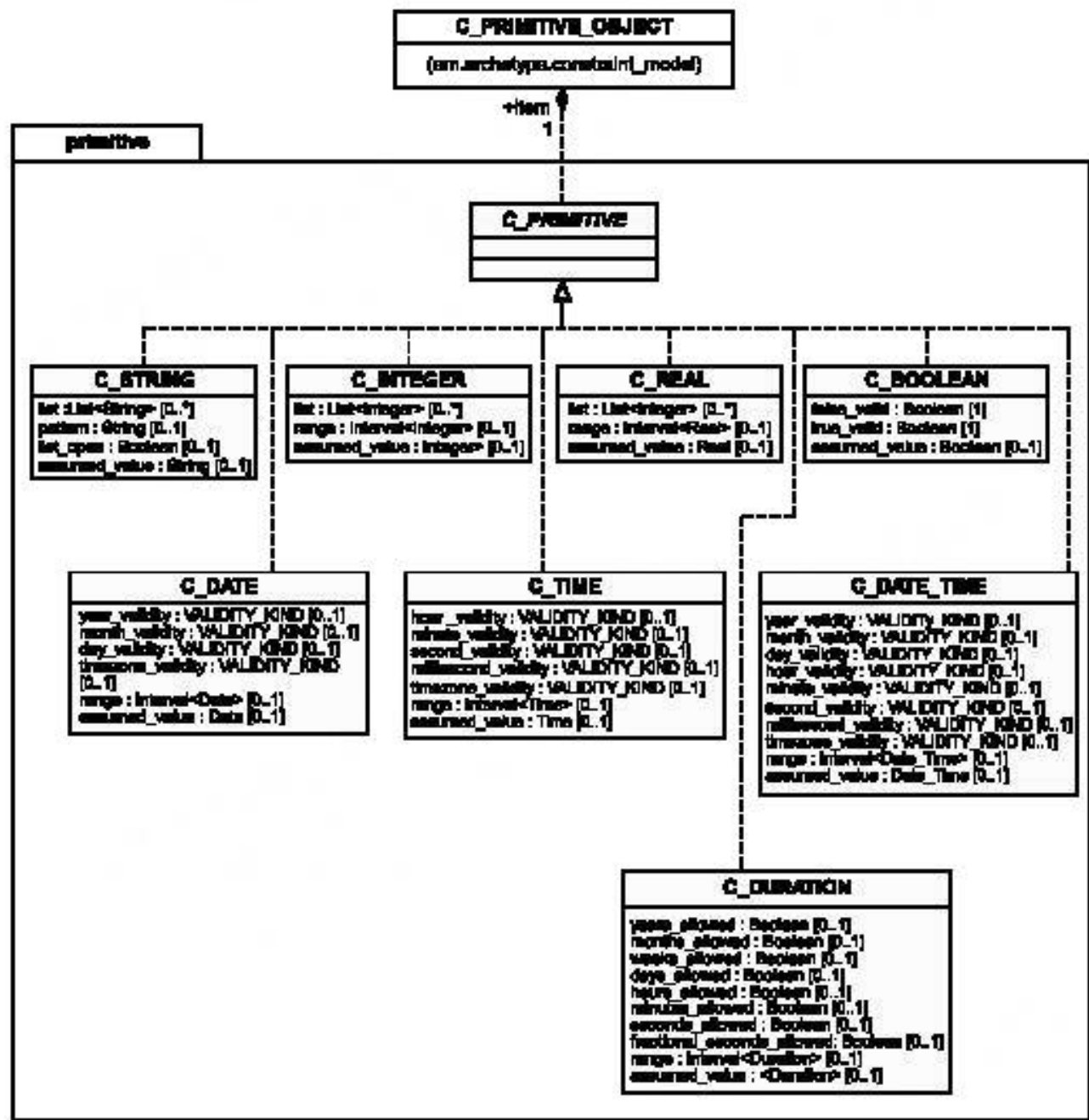
Рисунок 9 — Пакет primitive
