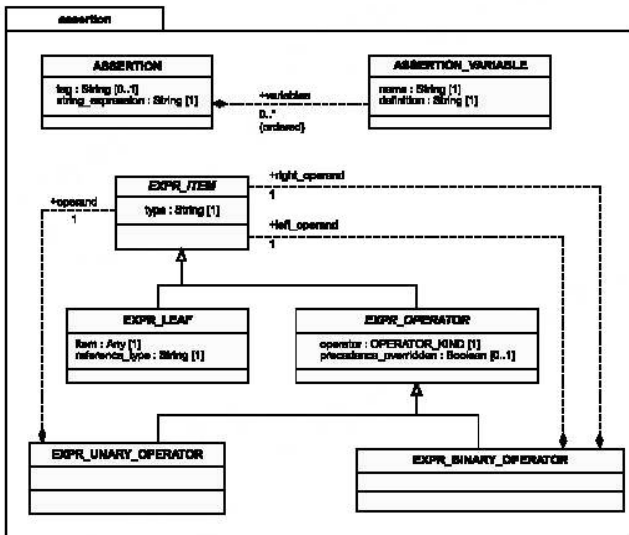
Рисунок 8 — Пакет assertion
