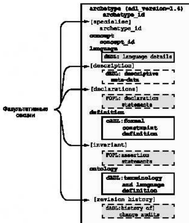
Рисунок 1 — Структура ADL-архетипа
