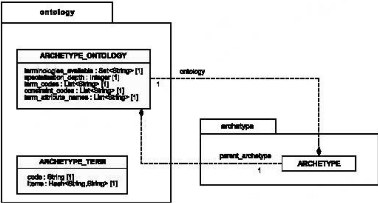
Рисунок 10 — Пакет ontology
