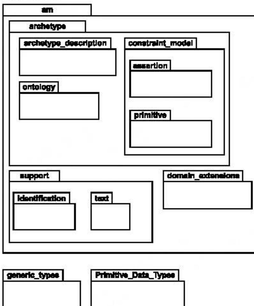
Рисунок 2 — Структура пакетов
