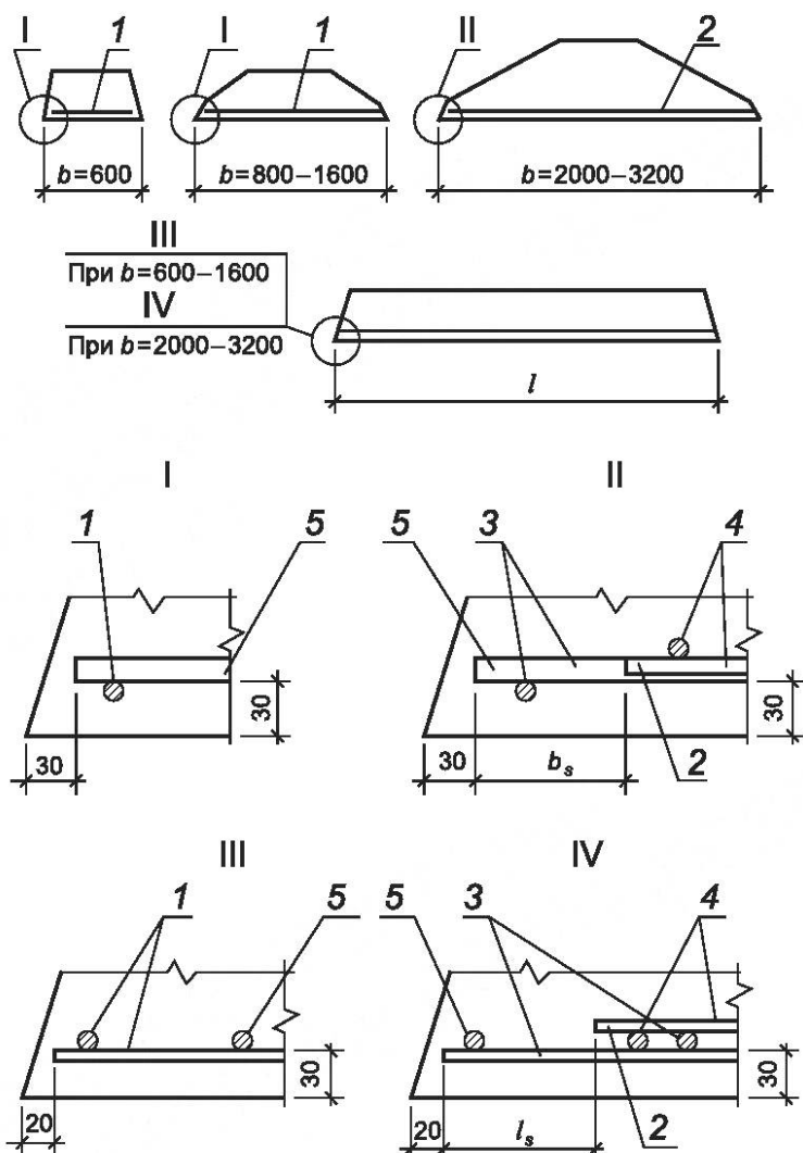
Рисунок 2 — Расположение арматурного блока и сеток в плите
