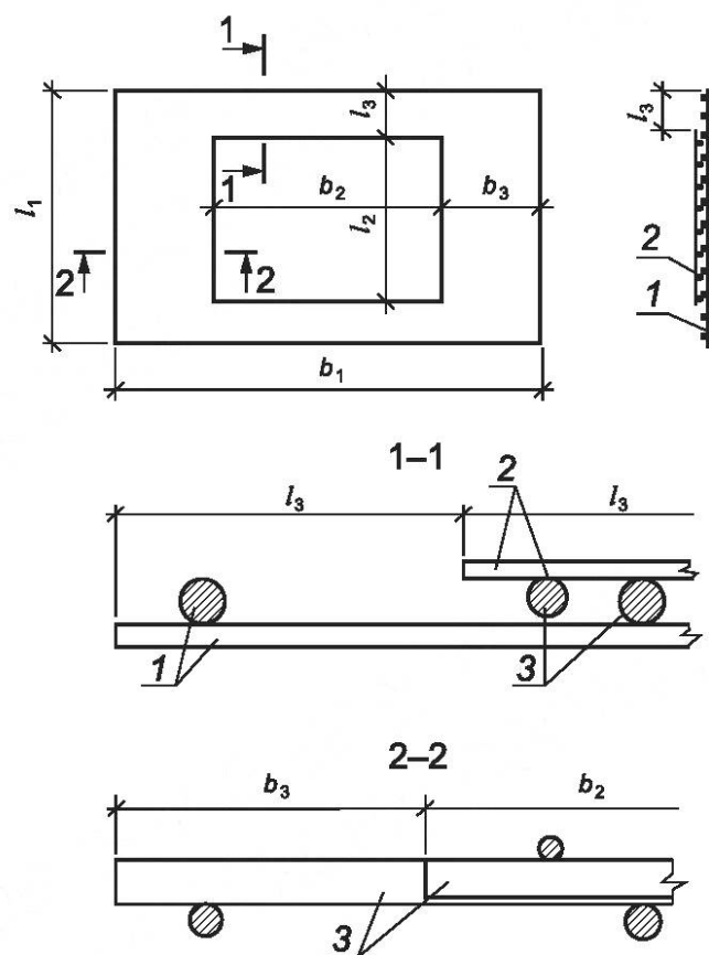
1 — нижняя сетка; 2 — верхняя сетка; 3 — рабочая арматура
