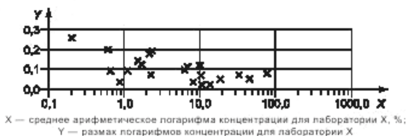
Рисунок 12 — Размах логарифмов концентраций повторных исследований лаборатории X
