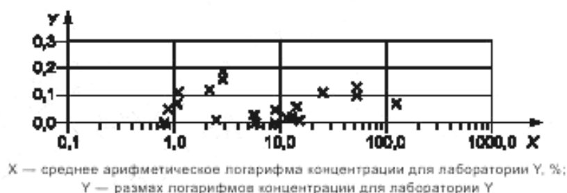
Рисунок 13 — Размах логарифмов концентраций повторных исследований лаборатории Y
