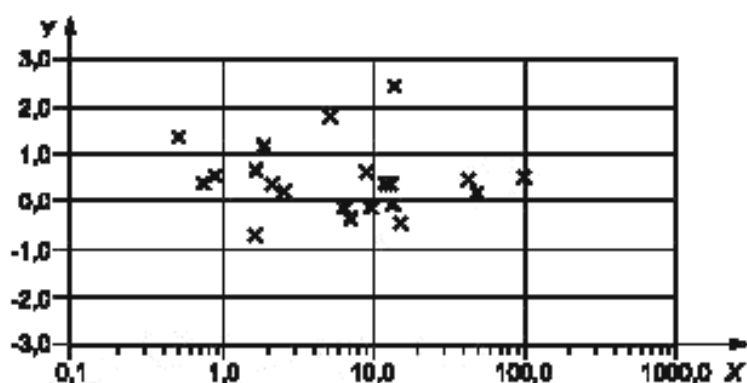
X — среднее арифметическое логарифма концентрации для лабораторий X и Y, %; Y — разность логарифмов концентрации для лаборатории Y и лаборатории X
