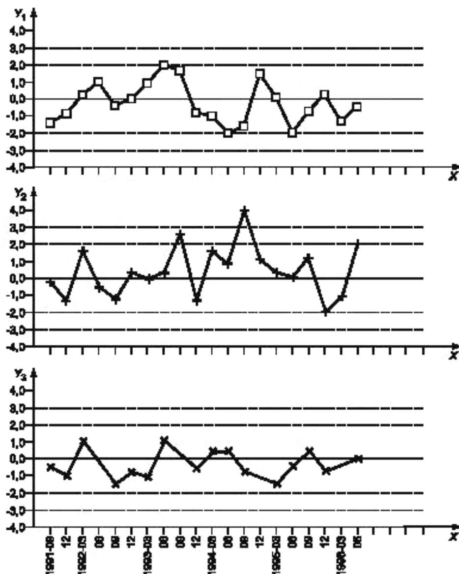
Рисунок 15 — Контрольные карты Шухарта для данных одной лаборатории в 20 раундах программы экспериментальной проверки компетентности (данные таблицы 16)
