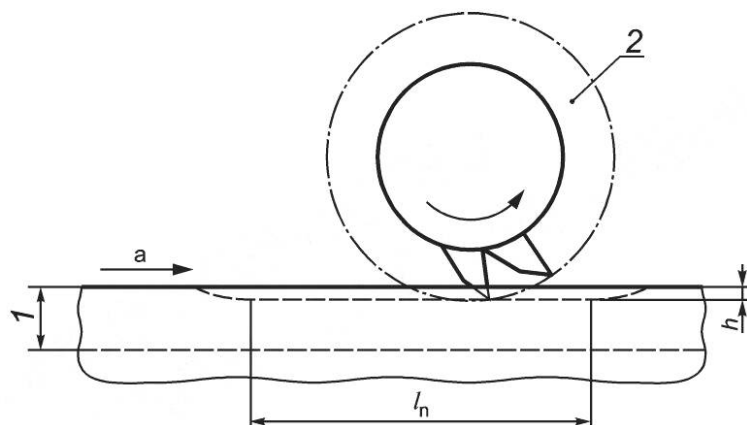
1 — стенка трубы; 2 — двусторонняя фреза с зубьями под углом 60°; h — глубина надреза, мм; l_n — длина надреза ( 1 \times d_n ) по центру испытательного образца; a — направление подачи образца
