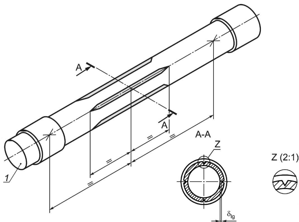
1 — концевая заглушка; \delta_{lg} — остаточная толщина, соответствующая 0,78—0,82 номинальной толщины стенки испытываемой трубы, мм
