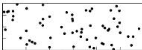
Рисунок А.6 — Пористость 4 %, 61 пора, d = 1 мм
