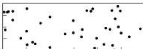
Рисунок А.4 — Пористость 2,5 %, 38 пор, d = 1 мм
