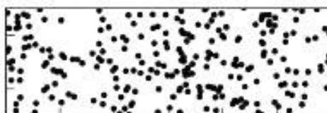
Рисунок А.9 — Пористость 16 %, 244 поры, d = 1 мм
