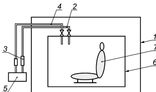
1 — термостат; 2 — кран-клапан; 3 — сорбционная трубка или картридж с ДНФГ; 4 — трубка из политетрафторэтилена (ПТФЭ); 5 — побудитель расхода; 6 — пластиковый мешок большого размера; 7 — деталь отделки салона АТС
