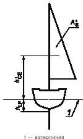
Рисунок 13 — Размеры h'_{CE} и h_{LP}
