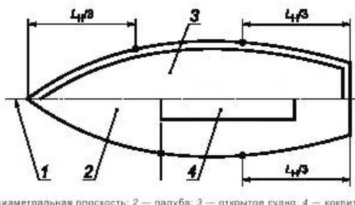
1 — диаметральной плоскости; 2 — палуба; 3 — открытое судно; 4 — кокпит
