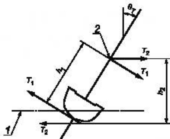
1 — ватерлиния; 2 — любое удобное место
