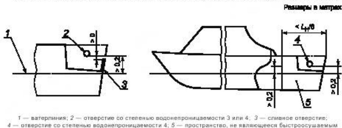
Рисунок 2 — Отверстия в нишах подвесного мотора
