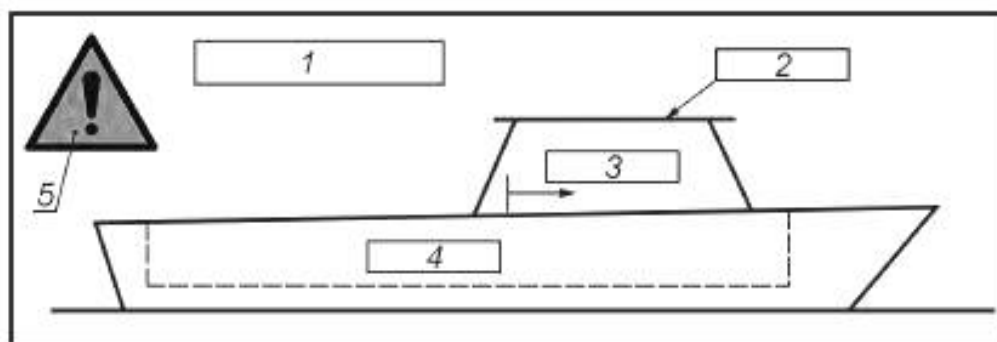
1 — текст, устанавливающий максимальное число людей на борту; 2 — текст, устанавливающий любые ограничения доступа, такие как «сидеть или стоять запрещено»; 3 — текст, устанавливающий любые ограничения доступа, такие как «максимальное число людей на палубе = 2»; 4 — текст, устанавливающий любые ограничения доступа, такие как «нет ограничений»; 5 — знак W001 «общее предупреждение» согласно ISO 7010
