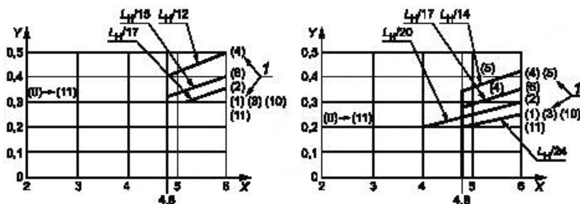
а) проектные категории А и В X — длина корпуса, м; Y — требуемая высота заливания, м, t — номера вариантов (см. таблицу 2)
