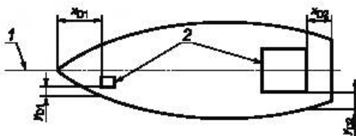
1 — диаметральной (осевой) линия; 2 — отверстия, считающиеся открытыми
