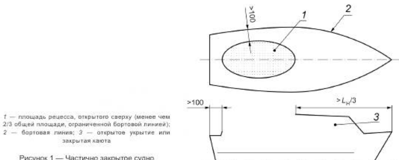
Рисунок 1 — Частично закрытое судно
