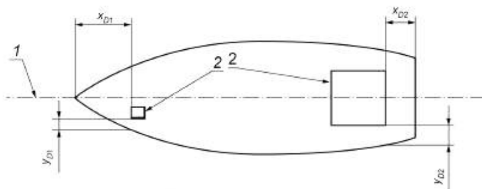
Рисунок А.1 — Размеры x_D и y_D
