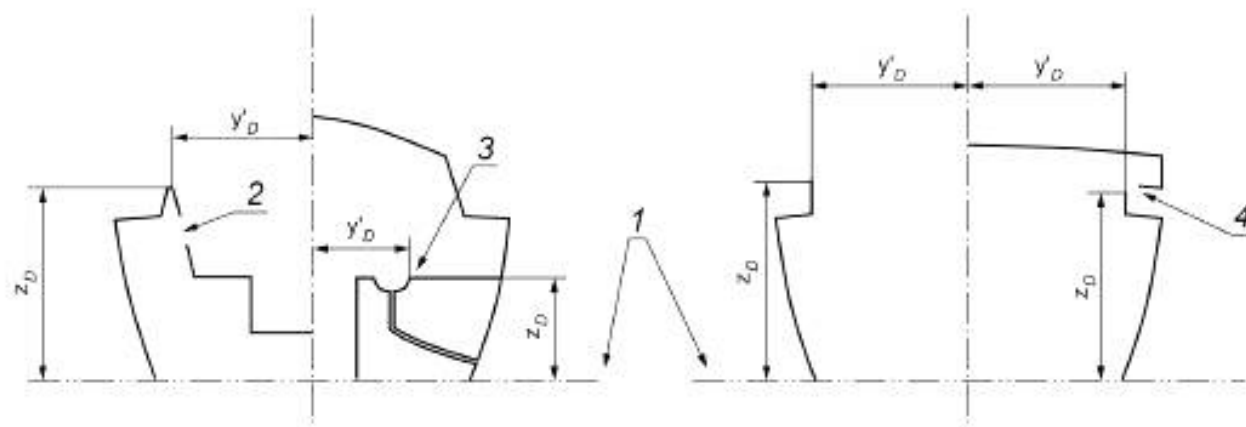
1 — ватерлиния; 2 — отверстия, считающиеся открытыми, защищенные коингом; 3 — пример внутреннего отверстия, считающегося открытым; 4 — пример воздухозаборника двигателя
