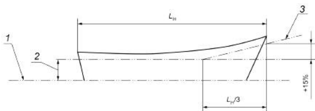
Рисунок 4 — Требуемая минимальная высота заливания — проектная категория D.
