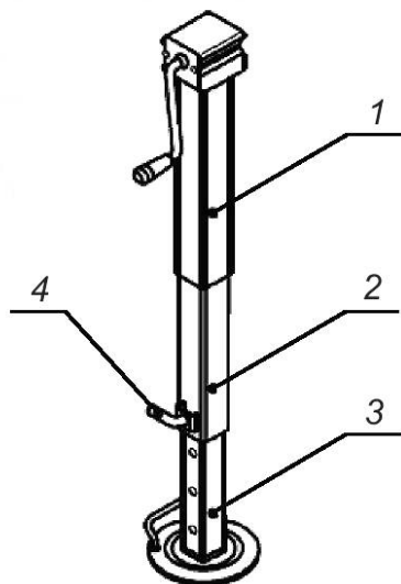
1 — внешняя труба (3.9); 2 — внутренняя труба (3.10); 3 — выдвижная опора (3.25); 4 — стопорный штифт
