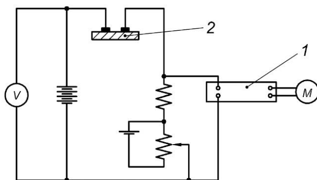
1 — усилитель постоянного тока; 2 — образец; V — вольтметр постоянного тока; M — вольтметр с индикацией Рисунок А.3 — Измерение тока с помощью усилителя постоянного тока
