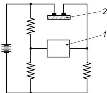
1 — детектор; 2 — образец
