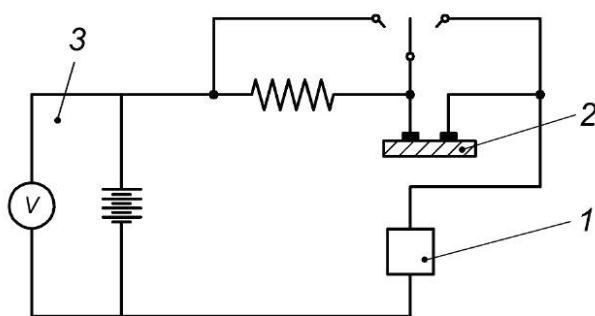
1 — микроамперметр или гальванометр с шунтом; 2 — образец; V — вольтметр постоянного тока (дополнительно)
