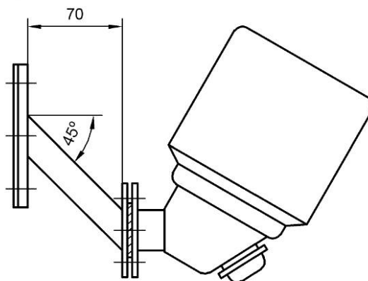
Рисунок 9 — Схема типового адаптера для клапана вдоха и выдоха для использования на испытательной установке при испытаниях самоспасателей
