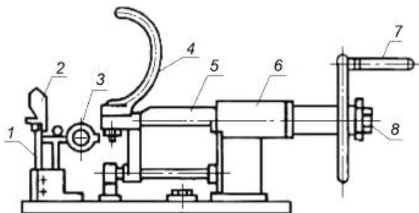
1 — силорезмерительная пружина; 2 — передний держатель; 3 — индикатор часового типа; 4 — задний держатель; 5 — подвижный шток; 6 — подшипник; 7 — ручной привод; 8 — ограничительная пробка
