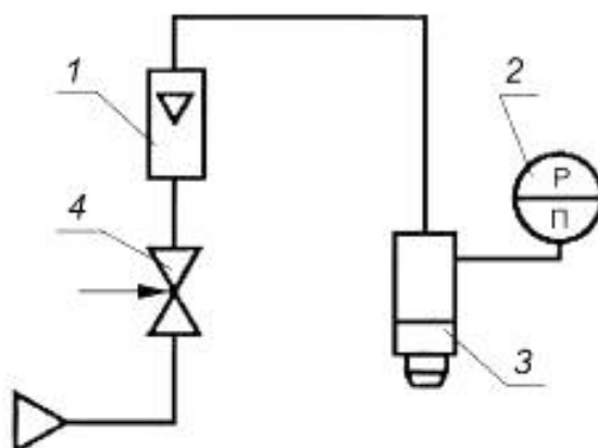
Рисунок 1 — Схема стенда для испытания сопротивления шлем-маски
