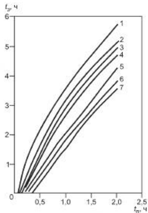
Рисунок Р.8 — Зависимость эквивалентной продолжительности пожара t_{э} от характерной продолжительности пожара t_n для железобетонных несущих стен
