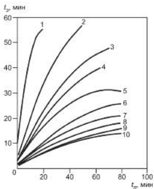
Рисунок Р.5 — Зависимость эквивалентной продолжительности пожара t_{э} от продолжительности пожара t_{п} для горизонтальных незащищенных металлических конструкций
