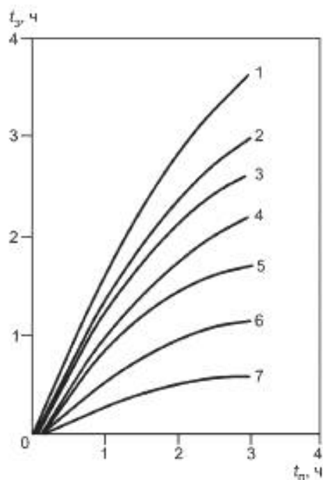
Рисунок Р.7 — Зависимость эквивалентной продолжительности пожара t_{э} от характерной продолжительности пожара t_n для огнезащищенных металлических и железобетонных конструкций перекрытия
