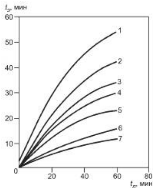
Рисунок Р.6 — Зависимость эквивалентной продолжительности пожара t_{э} от продолжительности пожара t_{п} для вертикальных незащищенных металлических конструкций
