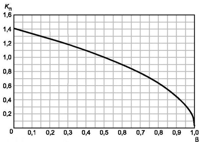
Рисунок Е.1 — Коэффициент K_n для несжимаемой жидкости
