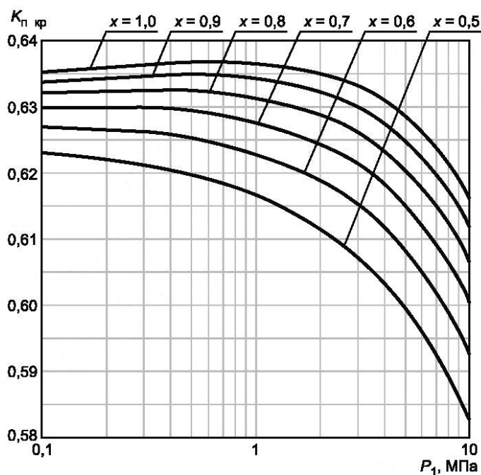
Рисунок Е.9 — Зависимость K_{п\text{кр}} = f(P_1) для влажного водяного пара
