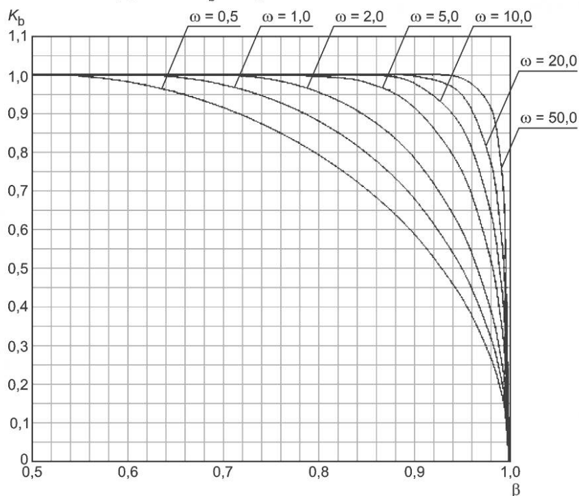
Рисунок Е.6 — Коэффициент K_b для омега-метода
