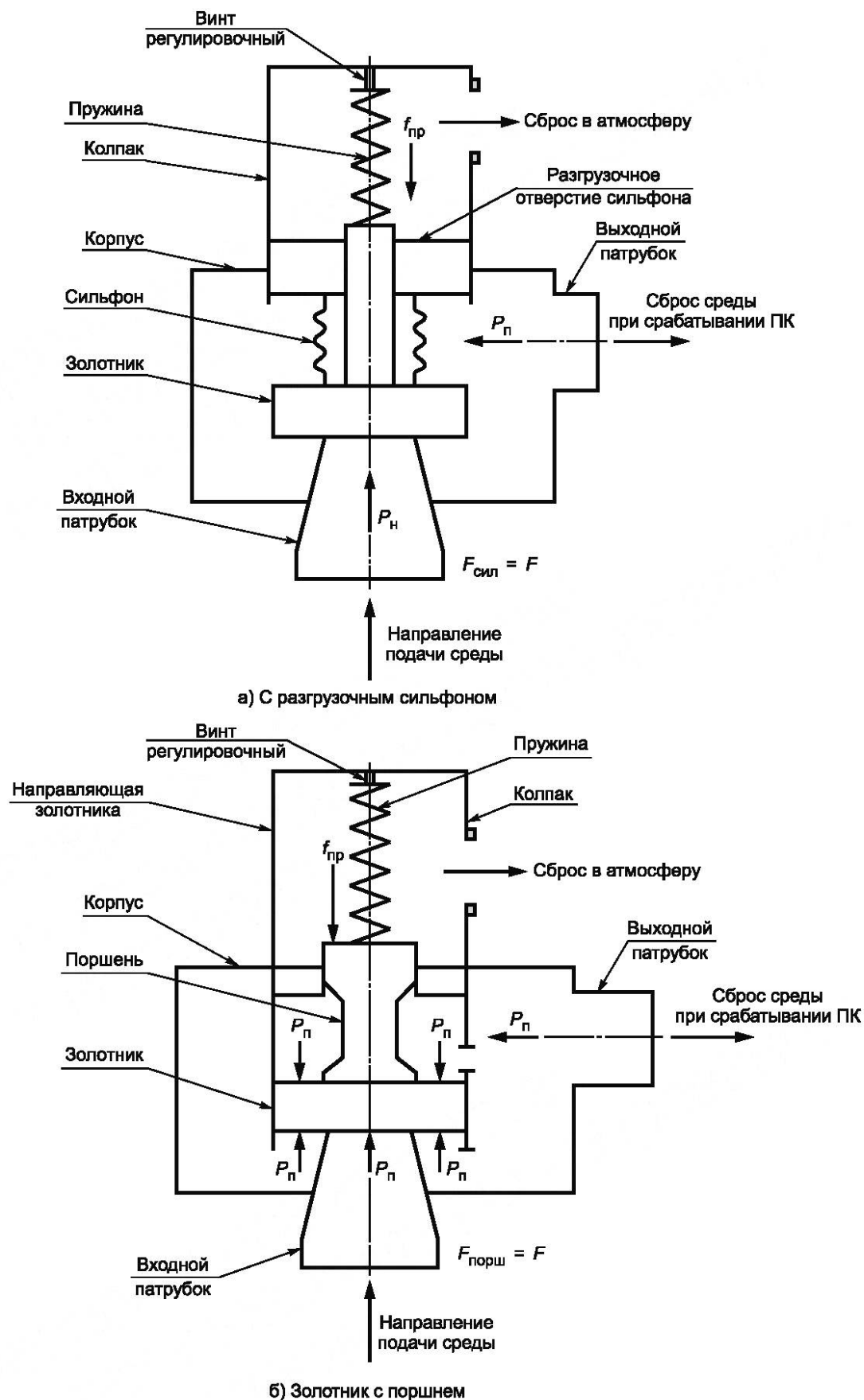
Рисунок В.2 — Статические давления в типовом разгруженном двухпозиционном ПК
