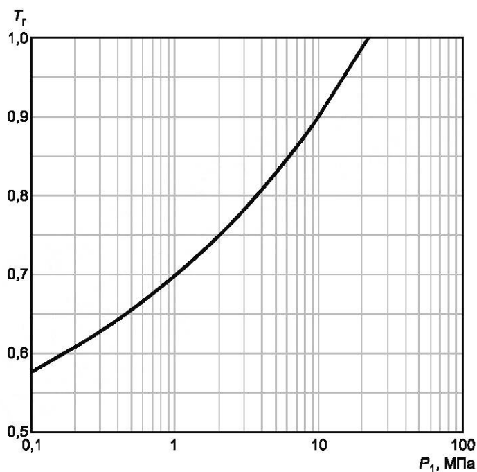
Рисунок Е.12 — Зависимость T_r = f(P_1) для насыщенных паров воды
