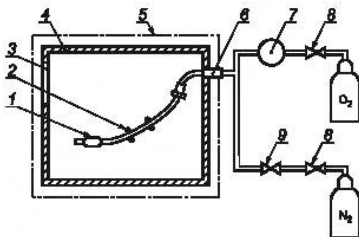
1 — тестируемая трахеальная трубка; 2 — опора трахеальной трубки с использованием двух хомутов; 3 — отверстие для доступа пучка лазерного излучения; 4 — защитный корпус (вид сбоку); 5 — крышка корпуса (может состоять из множества элементов); 6 — стопор обратного выброса; 7 — измеритель расхода кислорода и регулятор; 8 — регулятор давления с входными и выходными датчиками; 9 — быстродействующий клапан для инертного газа
