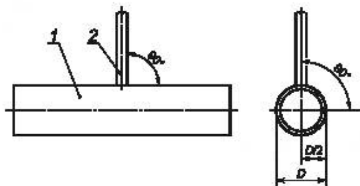
1 — тестируемый ствол; 2 — пучок лазерного излучения
