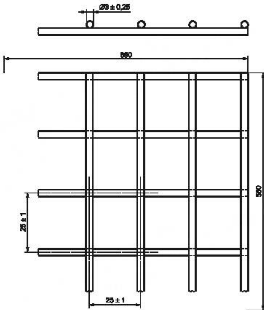
Рисунок 2 — Увеличенный дренажный экран
