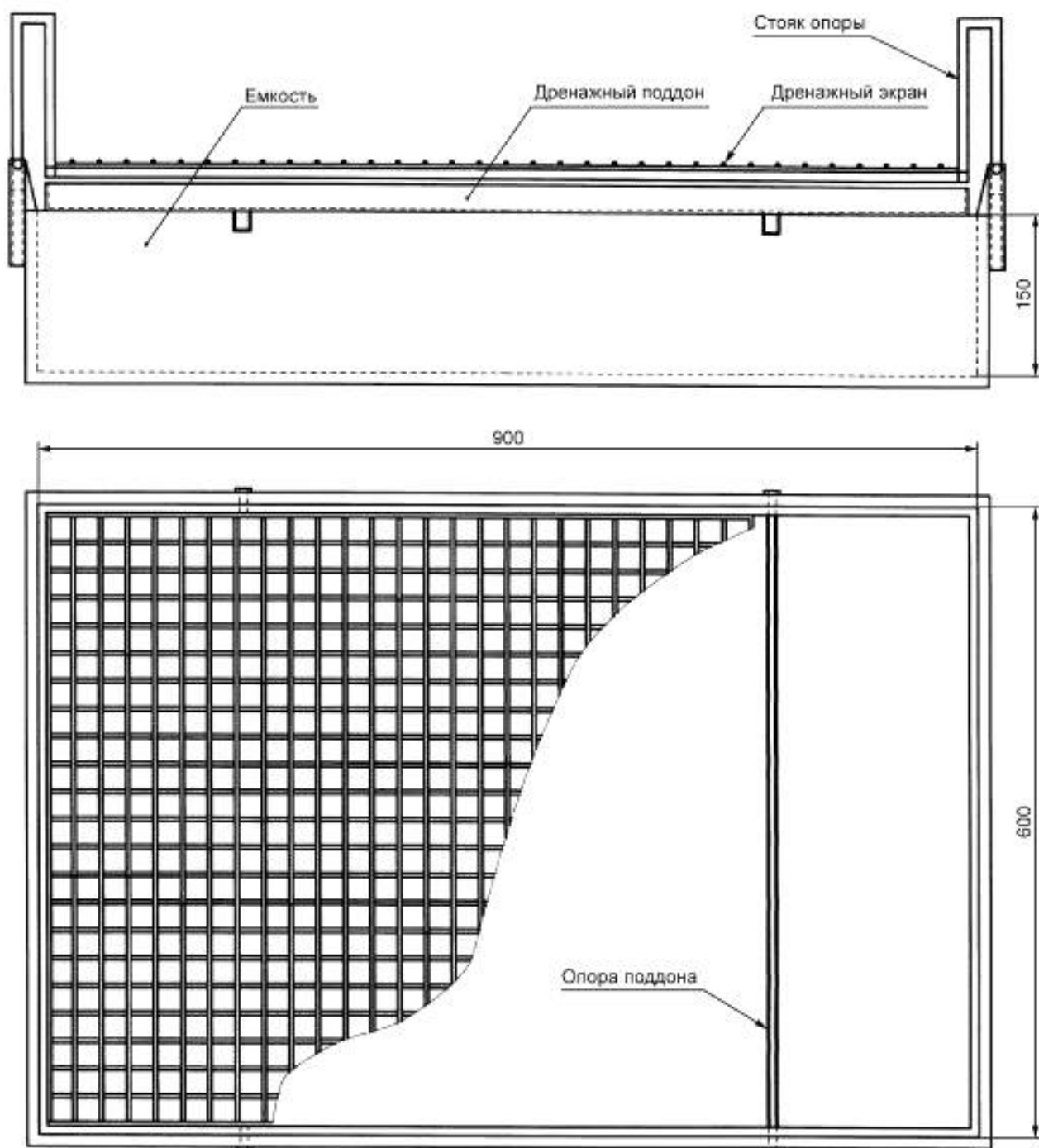
Рисунок 1 — Испытательное оборудование
