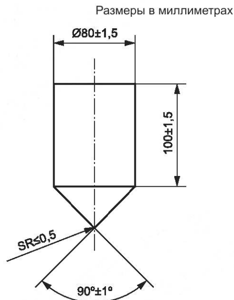
Рисунок 6 — Испытательный конус
