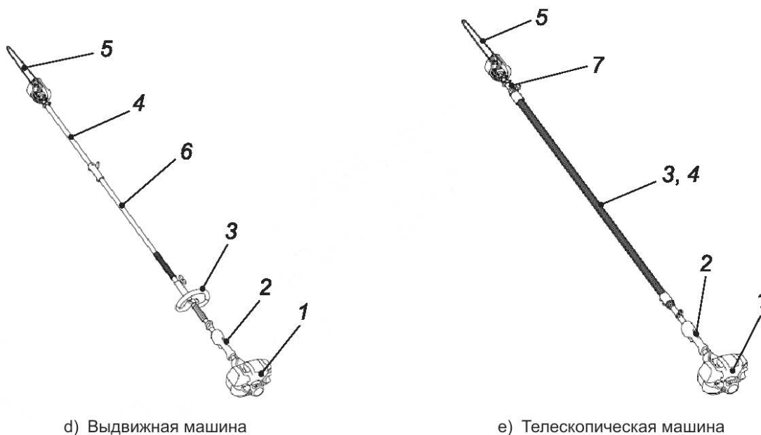
Рисунок 1 — Примеры механизированных секаторов на штанге со встроенным двигателем внутреннего сгорания
