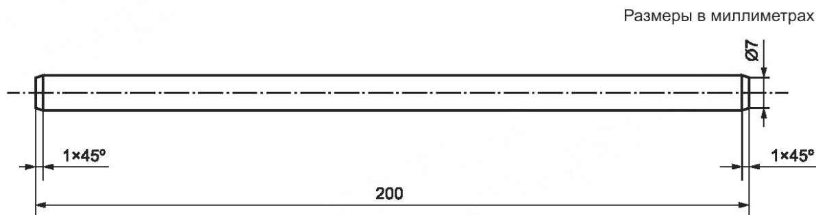
Рисунок В.1 — Тестовый щуп для проверки доступности линии подачи топлива
