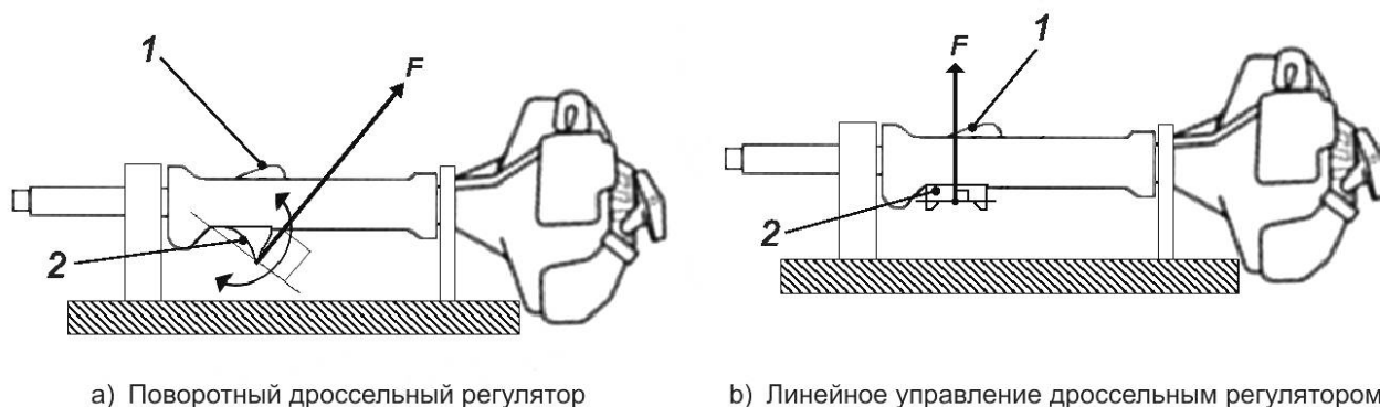
Рисунок 5 — Проверка работоспособности блокировки дроссельного регулятора
