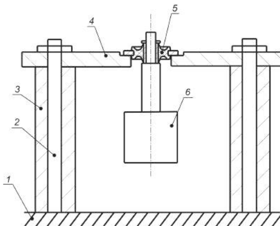
1 — рабочая платформа станда; 2 — копонка; 3 — ограничительная трубка; 4 — планка; 5 — амортизатор; 6 — груз
