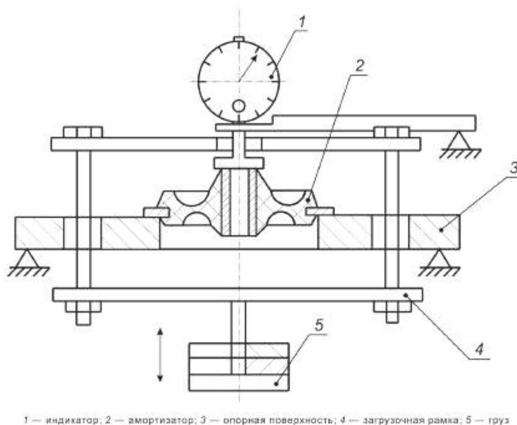
Рисунок Б.1 — Схема приспособления
