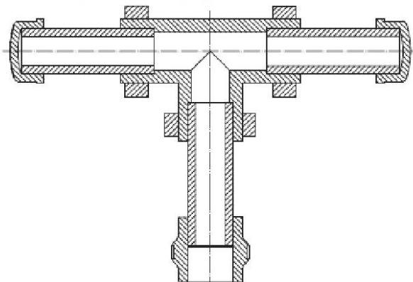
Рисунок 1 – Пример герметизации испытуемого образца с осевой нагрузкой, возникающей под действием гидростатического давления
