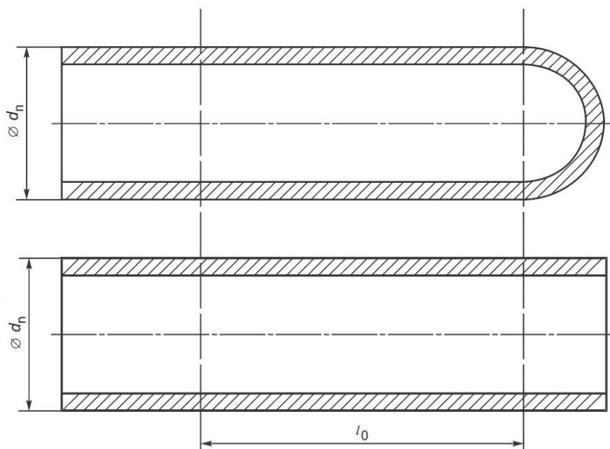
Рисунок 1 — Литьевые испытываемые образцы
