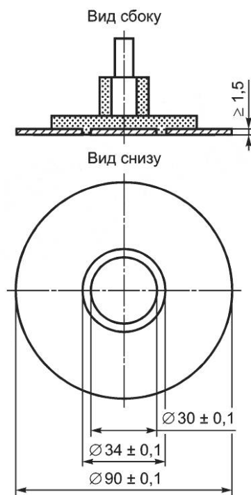
Рисунок 5 — Датчик для измерения поля
