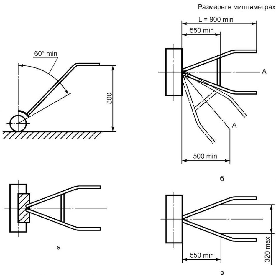
Рисунок 3 — Защита почвообрабатывающих органов переднего и ручного культиваторов
