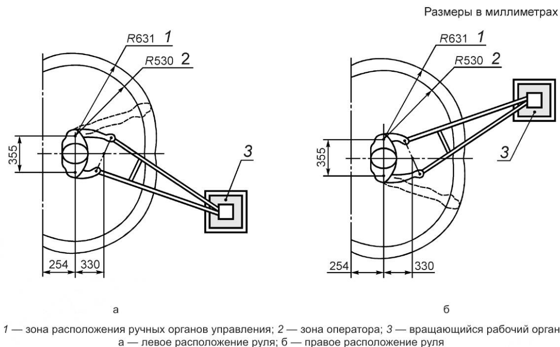
Рисунок 5 — Зона оператора, идущего рядом с культиватором
