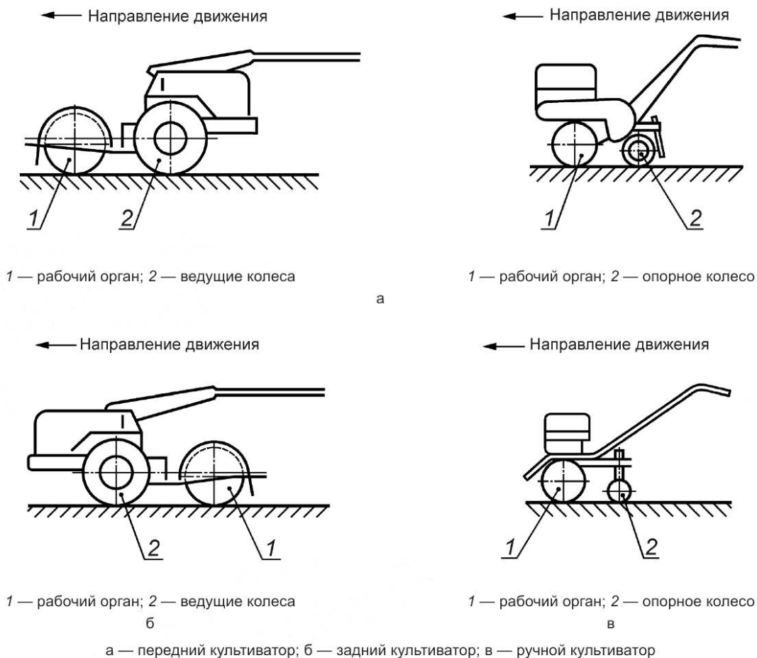
Рисунок 1 — Типы культиваторов
