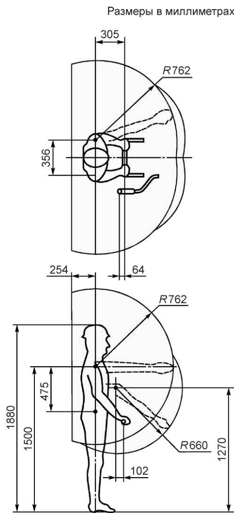
Рисунок 4 — Рабочая зона оператора
