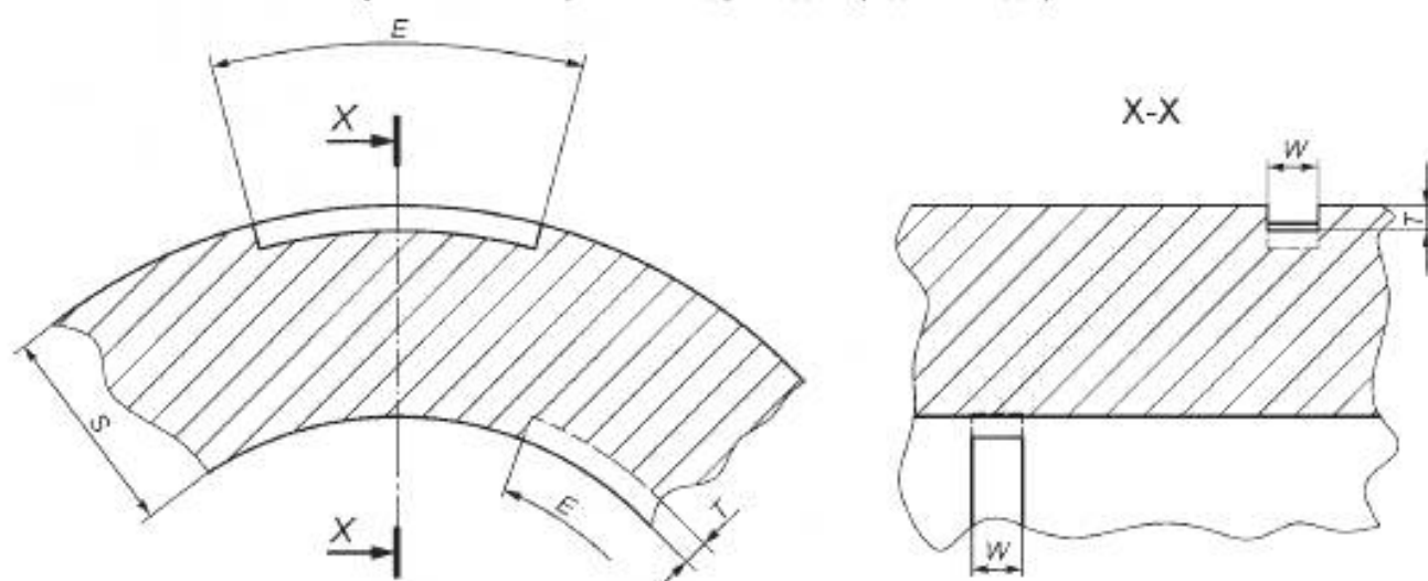
Рисунок В.1 — Контрольные надрезы для продольных дефектов
